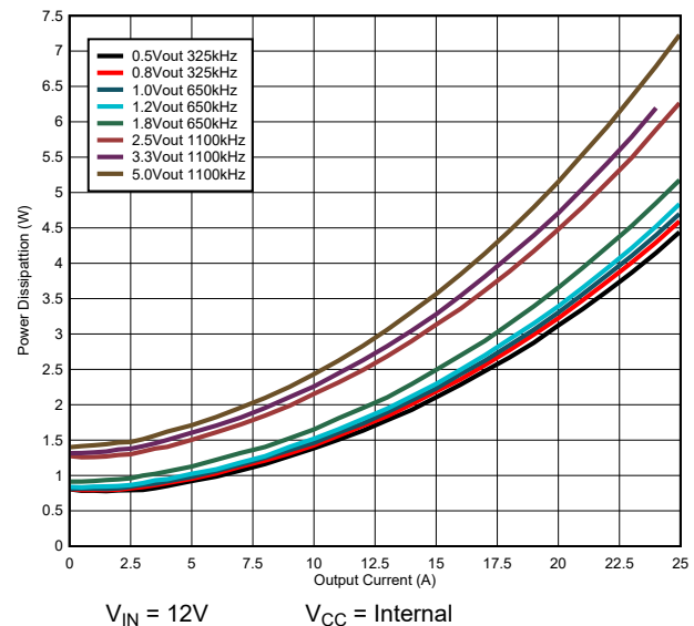
图 5-4. TPSM8S6B24 Power Dissipation vs Output Current
