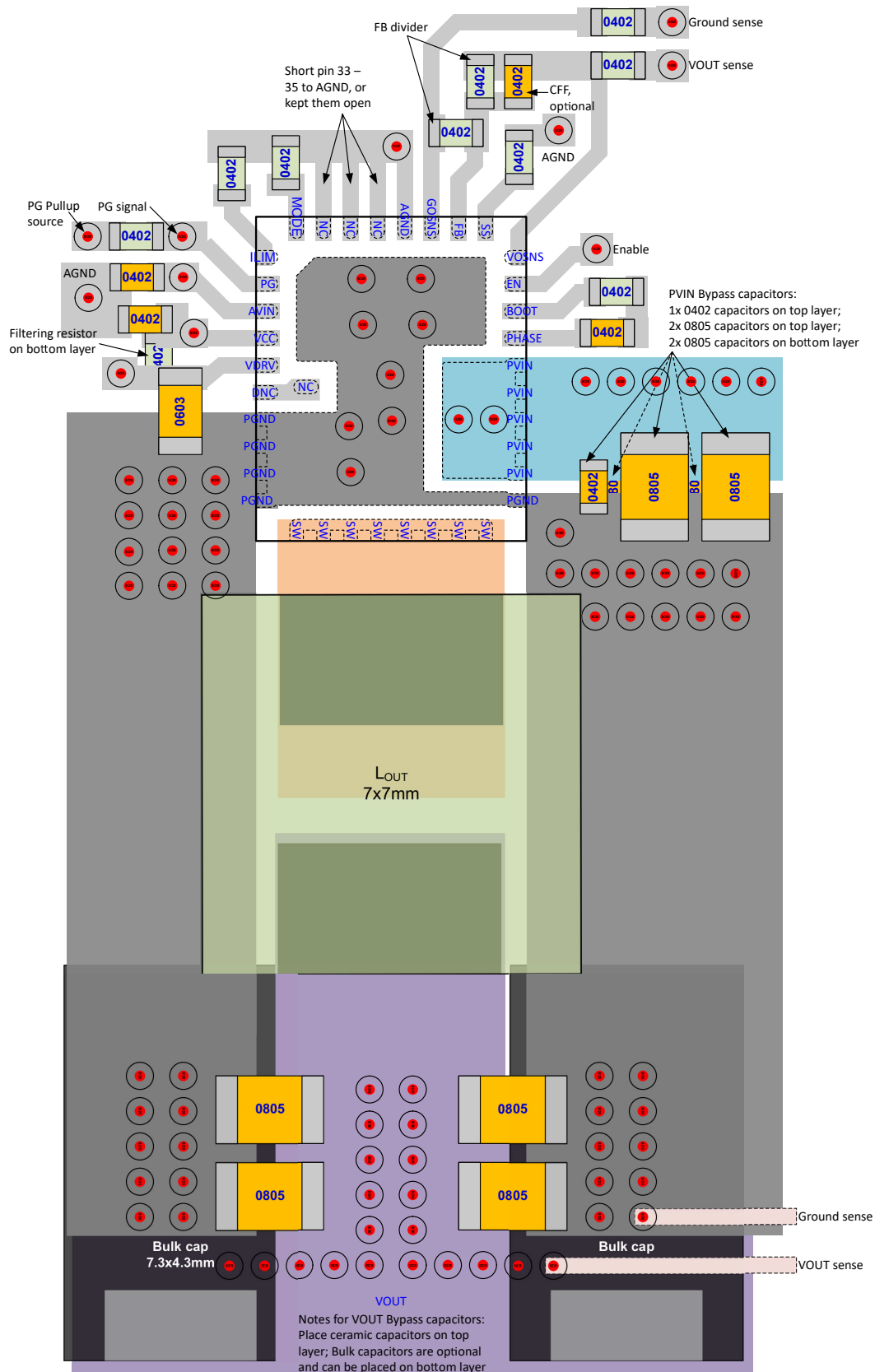
图 7-17. 布局建议
