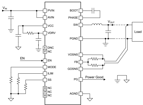
简化原理图
