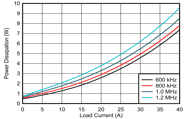
图 5-2. 功率损耗与输出电流间的关系
