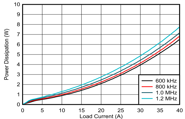
图 5-4. 功率损耗与输出电流间的关系
