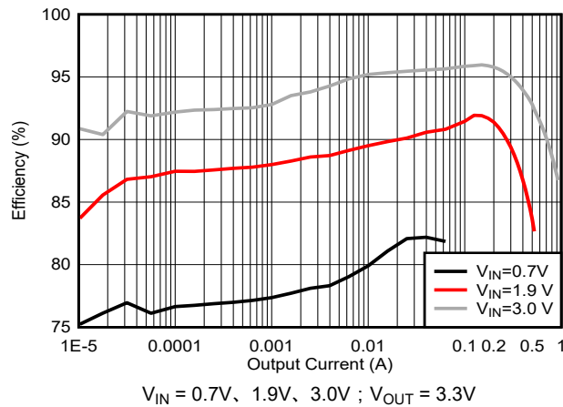
图 5-3. 不同输入电压在正常模式下的 3.3V VOUT 效率
