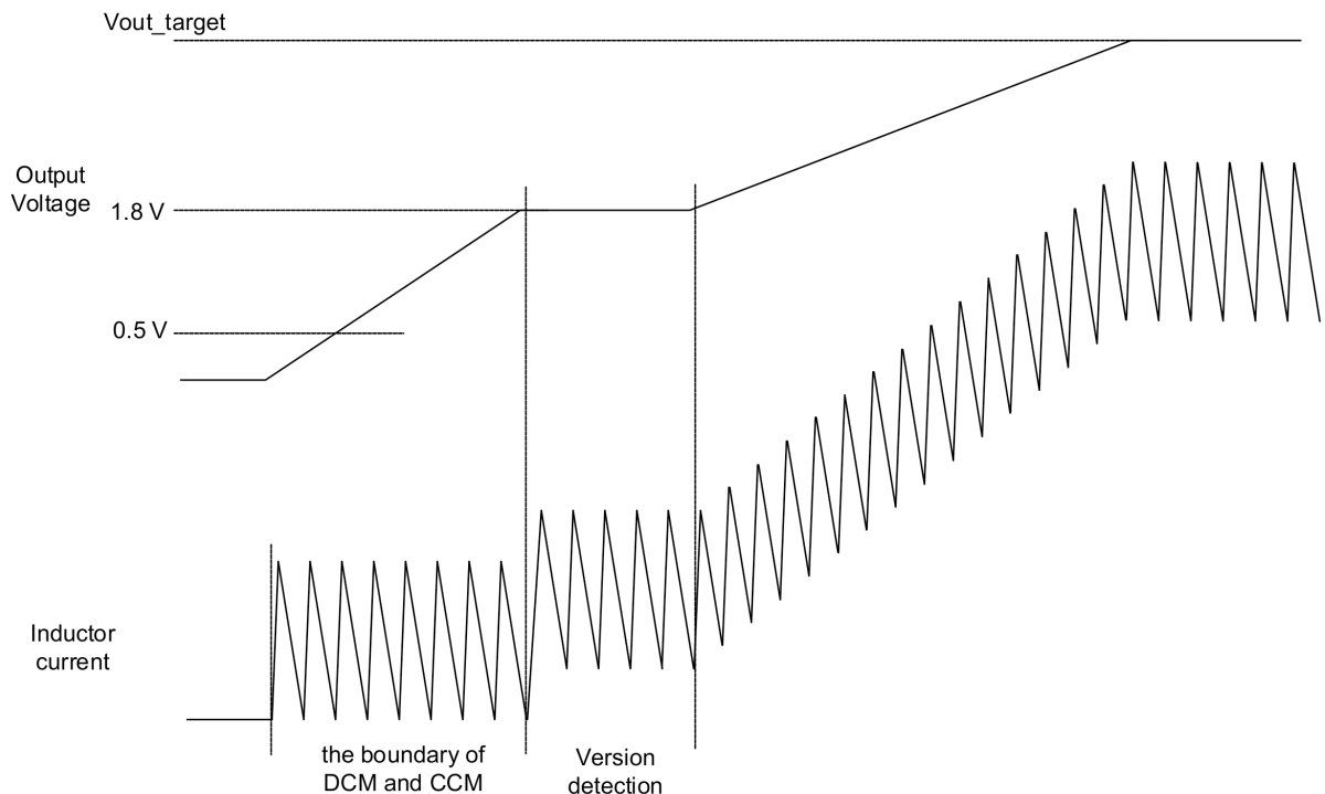
图 6-3. 软启动时序
