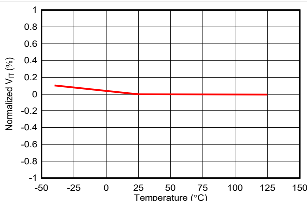
图 7-5. 标准化检测阈值电压 ( V_{IT} ) 与温度间的关系
