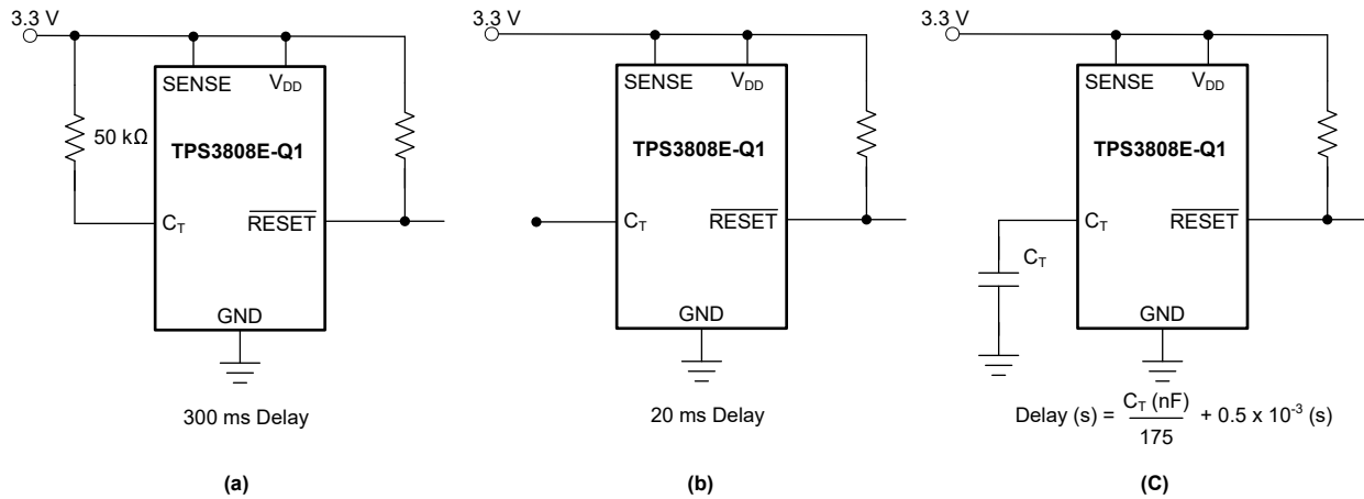
图 8-2. 用于设置 \overline{RESET} 延迟时间的配置
