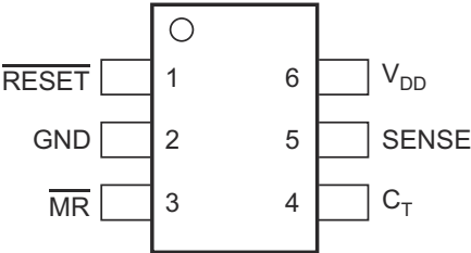
图 5-1. DBV 封装 6 引脚 SOT-23 顶视图
