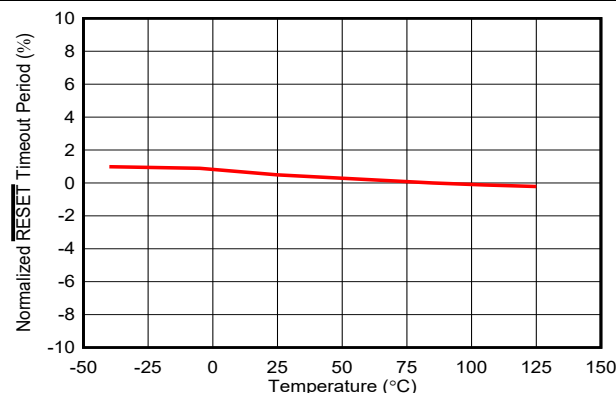
图 7-3. 标准化 RESET 超时周期与温度间的关系 ( C_T = 开路, C_T = V_{DD} , C_T = 任意)
