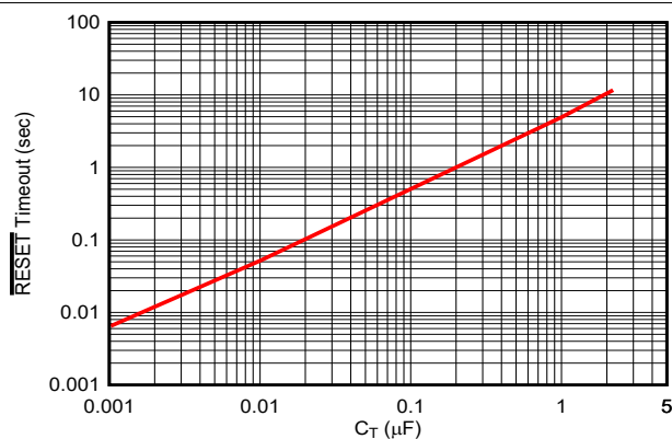
图 7-2. RESET 超时周期与 C_T 间的关系
