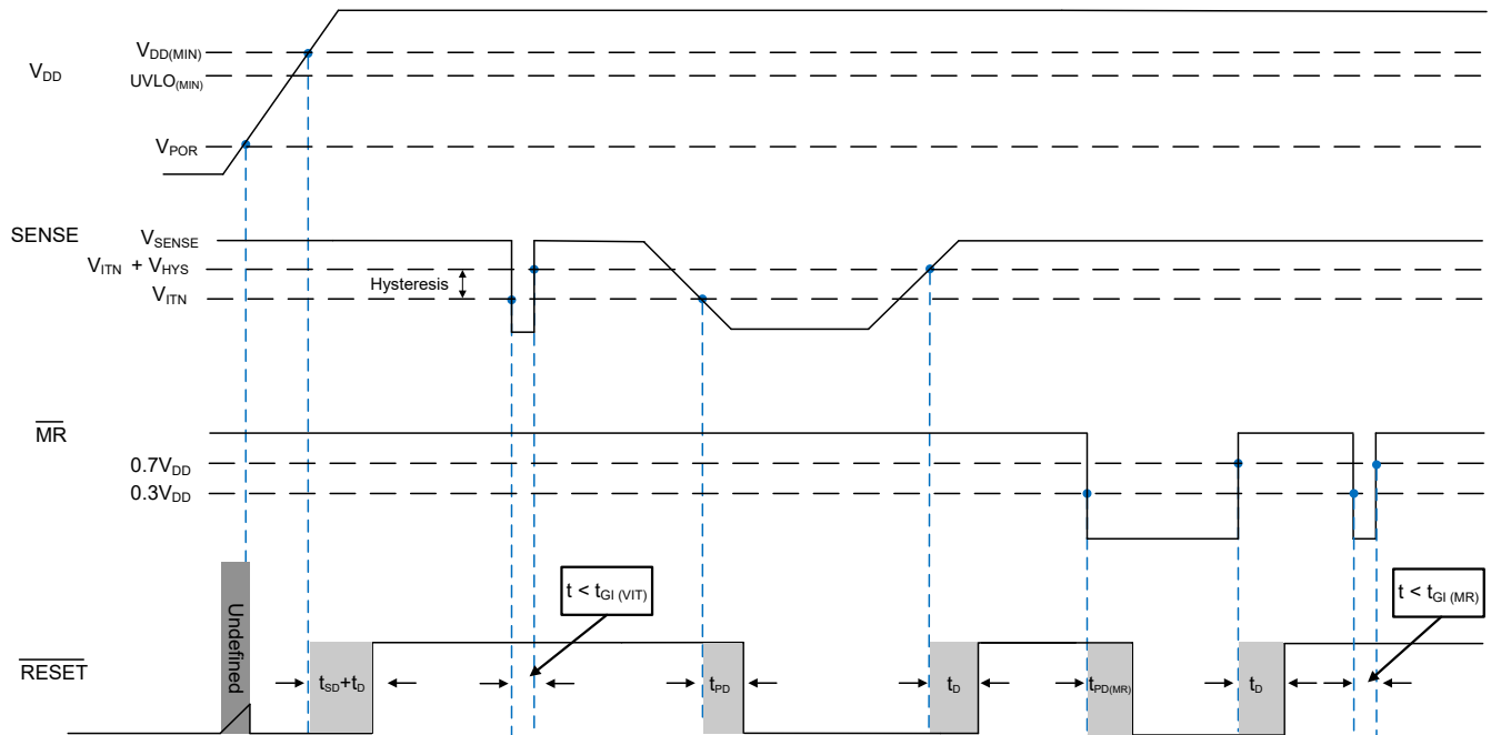
图 6-1. 时序图
