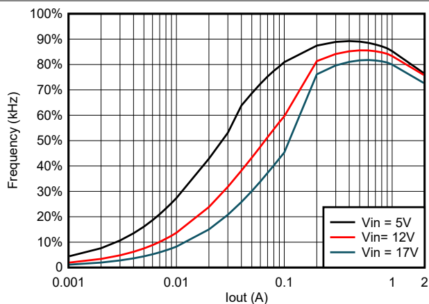
图 5-11. TPS562206 在 0.6Vout 且使用 1.5uH 电感器时的效率
