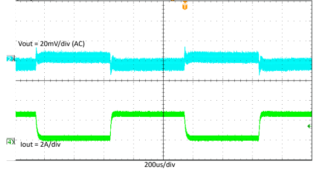
图 7-21. TPS562206 电流为 0A 至 2A 时的负载瞬态
