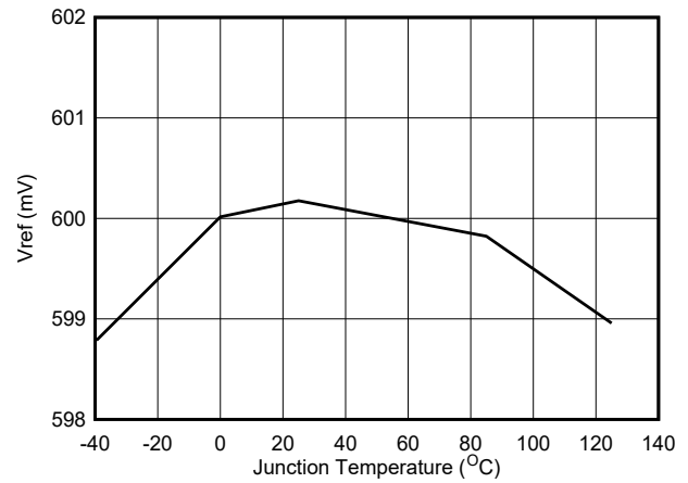
图 5-2. Vref 电压
