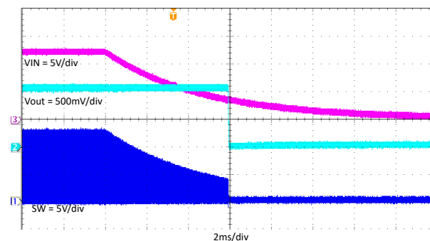
图 7-17. TPS562203 在负载电流为 2A 时断电
