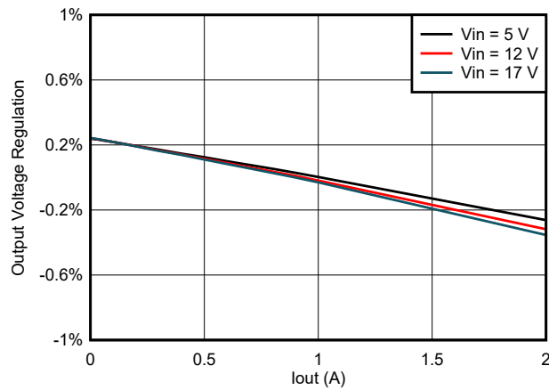
图 7-4. TPS562203 负载调整率与负载间的关系
