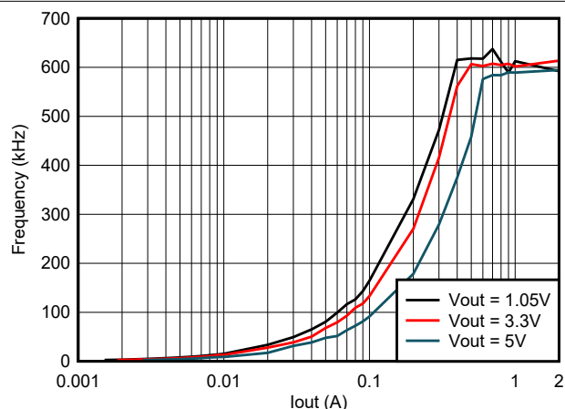
图 5-8. TPS562203 频率与负载间的关系
