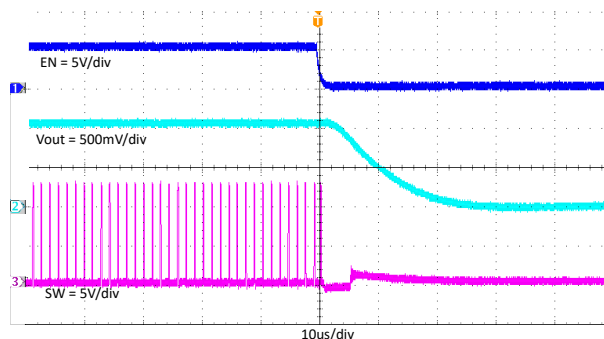
图 7-15. TPS562206 在负载电流为 2A 时使能关
