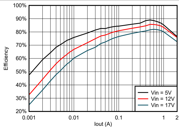
图 5-10. TPS562203 在 0.6Vout 且使用 1.5uH 电感器时的效率
