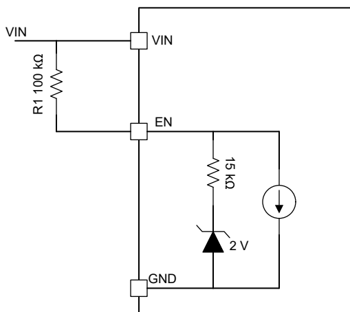
图 6-1. EN 块电路
