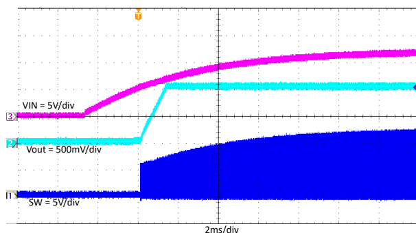
图 7-16. TPS562203 在负载电流为 2A 时上电
