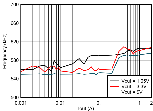
图 5-9. TPS562206 频率与负载间的关系
