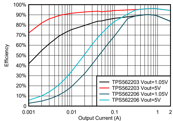
TPS562203 和 TPS562206 效率
