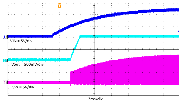
图 7-18. TPS562206 在负载电流为 2A 时上电
