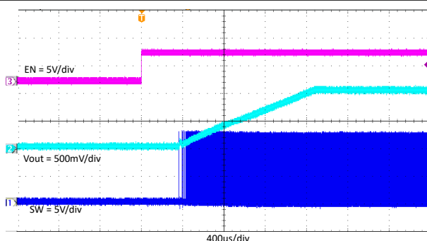
图 7-12. TPS562203 在负载电流为 2A 时使能开
