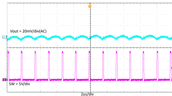
图 7-9. TPS562206 输出电压纹波 (0.1A 负载)
