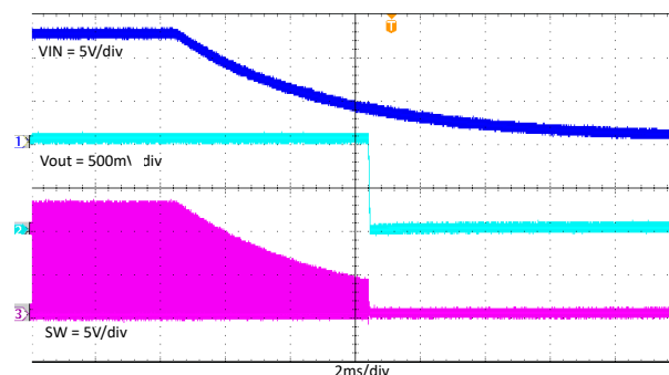
图 7-19. TPS562206 在负载电流为 2A 时断电
