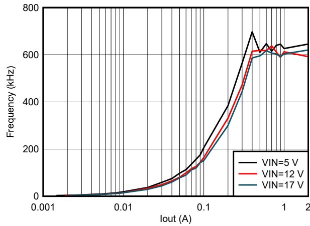
图 7-2. TPS562203 频率与负载间的关系
