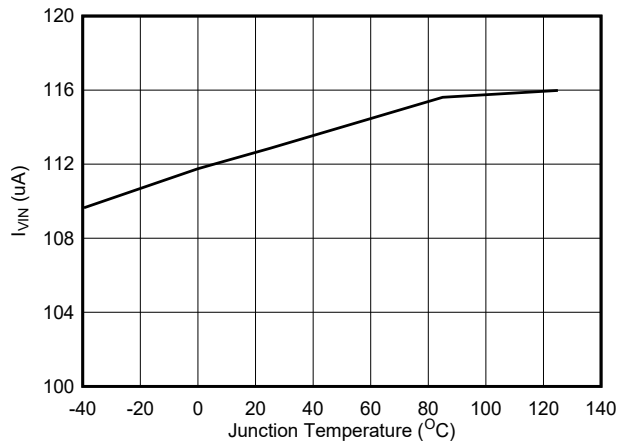
图 5-1. TPS562203 静态电流
