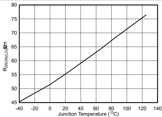
图 5-5. 低侧 R_{dson}
