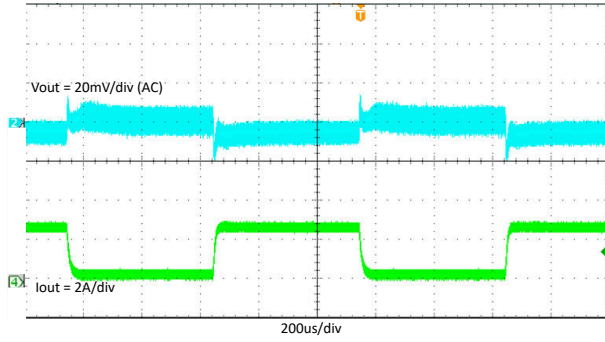
图 7-20. TPS562203 电流为 0A 至 2A 时的负载瞬态
