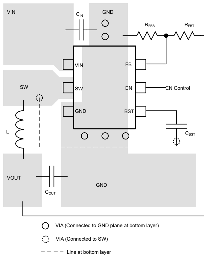
图 7-22. TPS562203 布局
