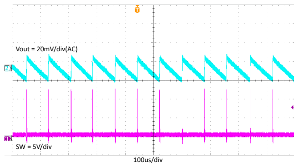
图 7-8. TPS562203 输出电压纹波 (0.1A 负载)
