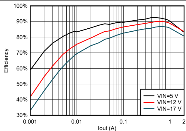
图 5-12. TPS562203 在 1.05Vout 且使用 2.2uH 电感器时的效率
