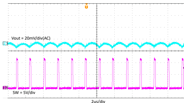
图 7-10. TPS562203 输出电压纹波 (2A 负载)
