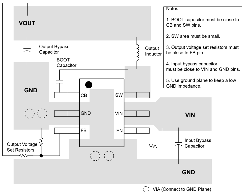
图 8-10. 布局
