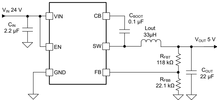
图 8-1. 应用电路
