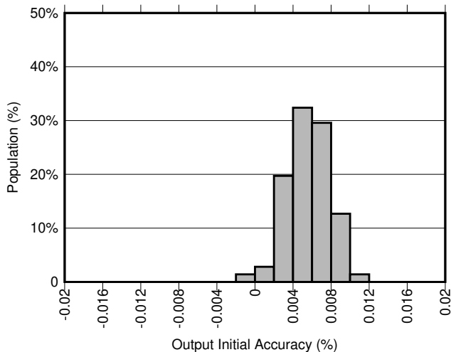
图 6-3. 精度分布
