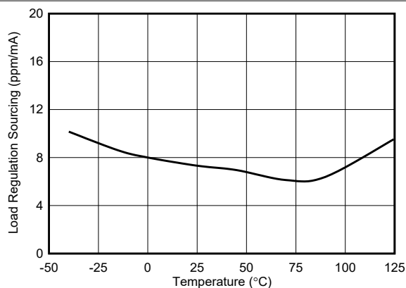
图 6-5. 负载调整率 (拉电流) 与温度间的关系
