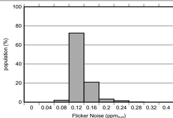
图 7-5. 0.1Hz 至 10Hz 电压噪声 (C NR = 100 μF)
