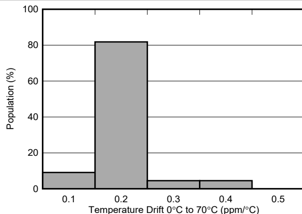
图 6-2. 漂移分布
