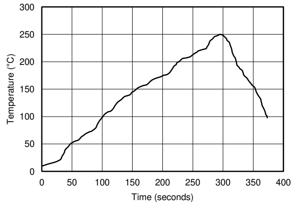
图 7-12. 回流焊曲线
