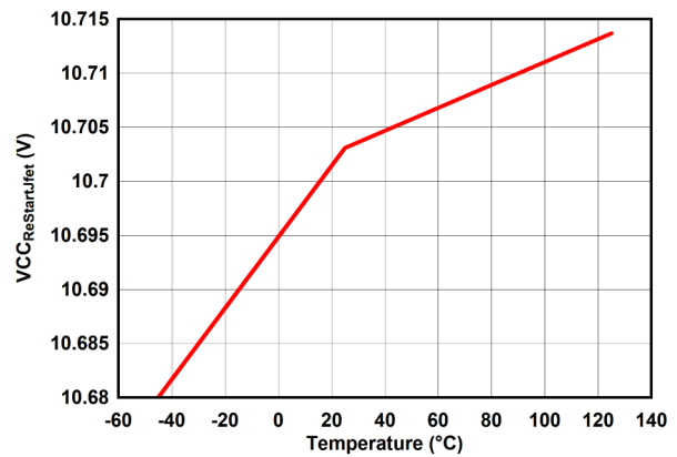
图 6-22. V_{\text{CC\_ReStartJfet}} 与温度间的关系
