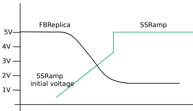
图 7-15. 软启动运行
