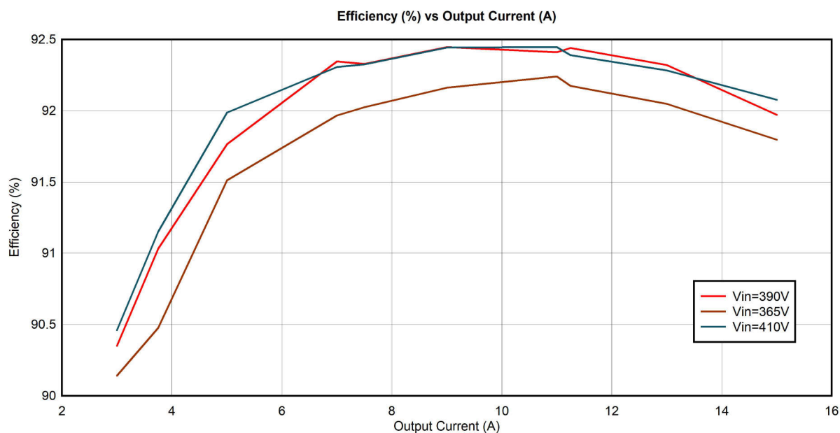
图 8-3. 效率
