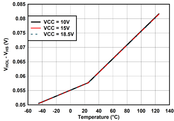
图 6-19. ( V_{\text{HOL}} - V_{\text{HS}} ) 与温度间的关系
