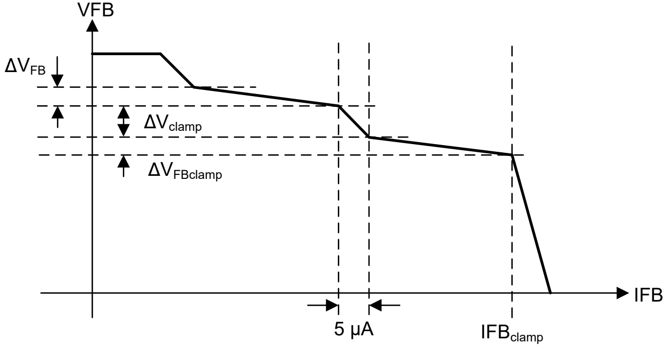
图 7-5. FB 引脚电压与 FB 引脚电流间的关系
