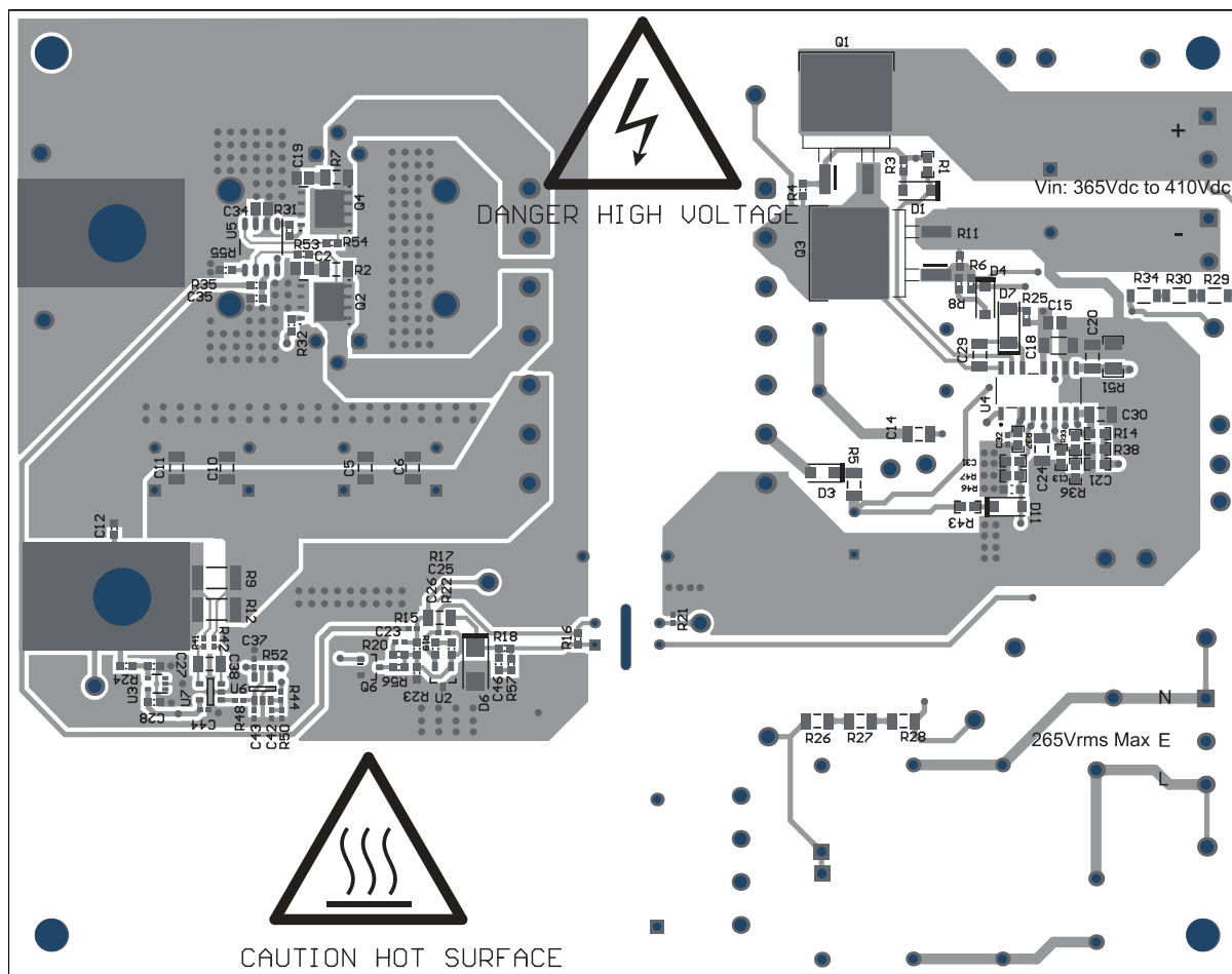
图 8-8. UCC25660EVM-064 ( 底视图 )
