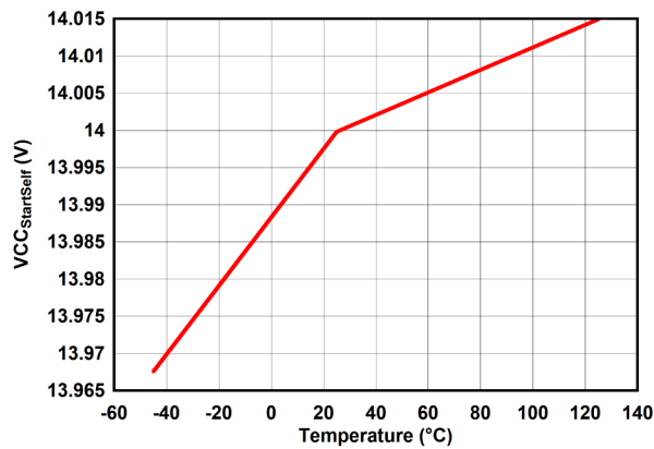
图 6-21. V_{\text{CC\_StartSelf}} 与温度间的关系
