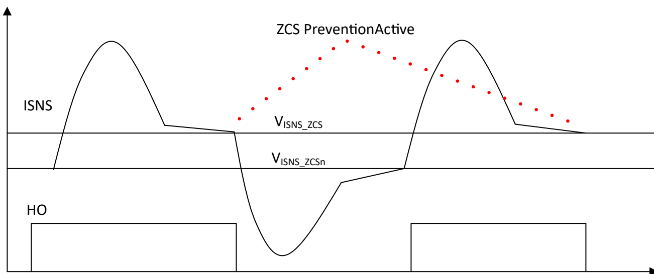
图 7-8. ZCS 保护
