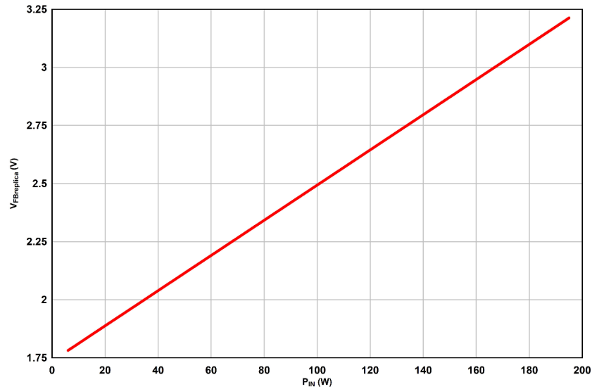
图 8-2. FB\text{replica} 与 P_{in} 间的关系
