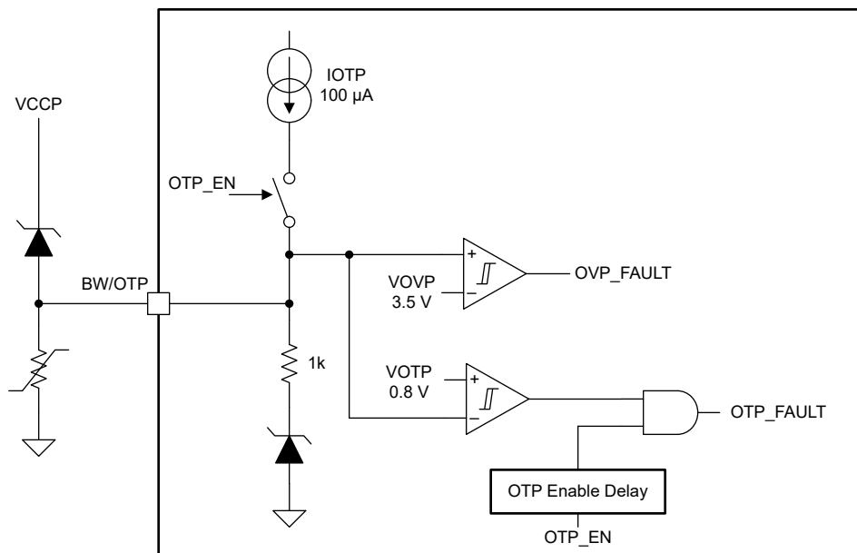
图 7-7. mOVP/OTP 保护架构
