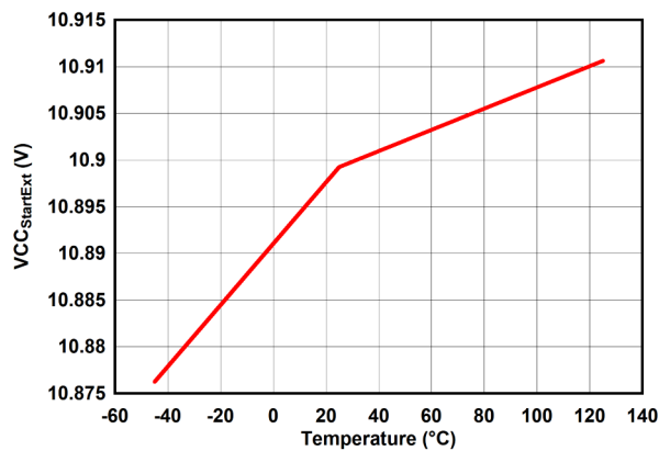
图 6-23. V_{\text{CC\_StartExt}} 与温度间的关系
