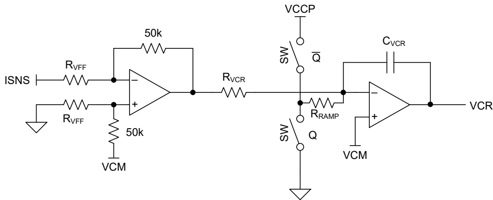
图 7-3. VCR 合成器方框图
