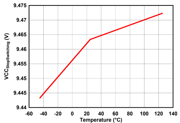
图 6-24. V_{\text{CC\_StopSwitching}} 与温度间的关系
