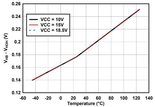
图 6-20. ( V_{\text{HB}} - V_{\text{HOH}} ) 与温度间的关系
