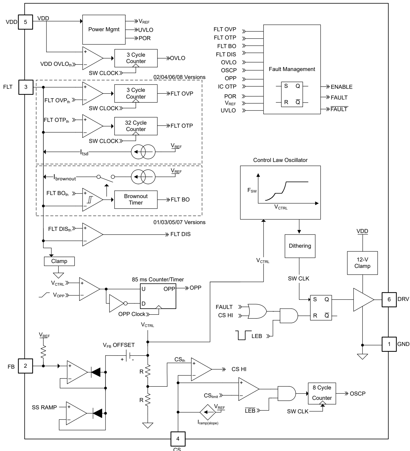
图 7-2. 功能方框图
