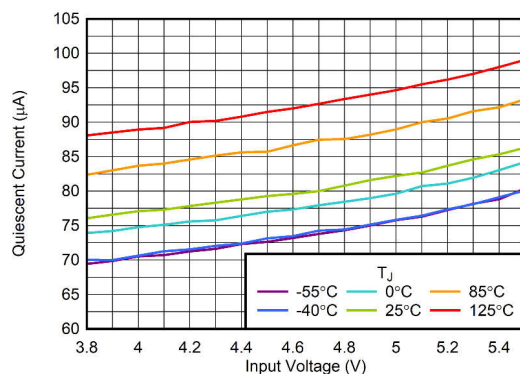
图 5-6. 静态电流与 V_{IN} 间的关系
