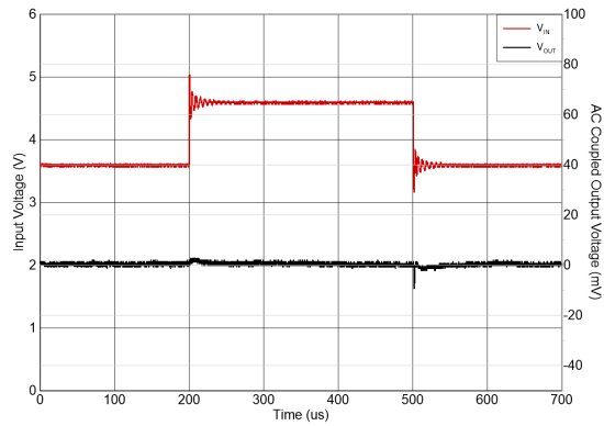
图 5-13. 线路瞬态
