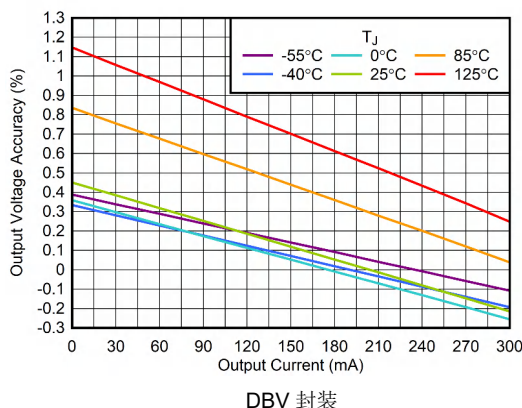
图 5-4. 输出电压精度与 I_{OUT} 间的关系
