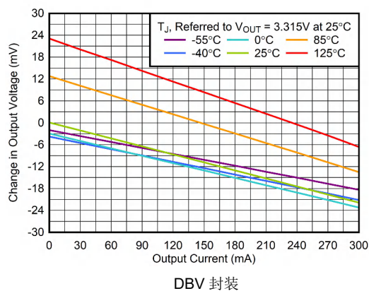
图 5-2. 负载调整率与 I_{OUT} 间的关系
