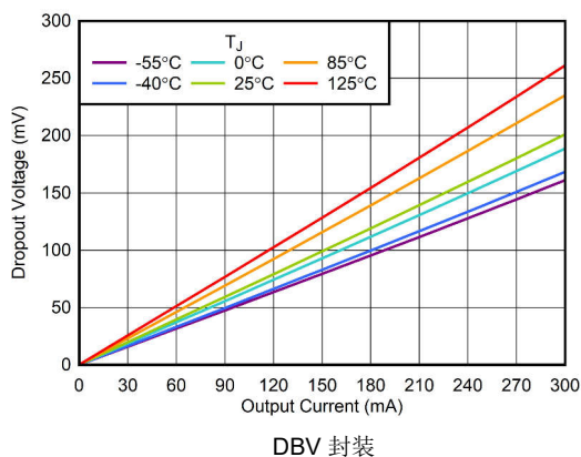
图 5-5. 压降与 I_{OUT} 间的关系
