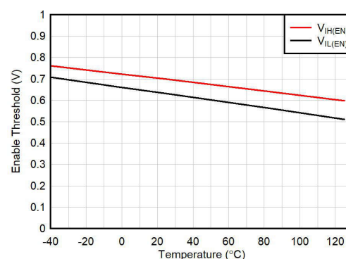
图 5-10. 使能逻辑阈值与温度间的关系
