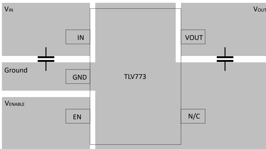
图 7-4. DBV 封装 (SOT-23) 典型布局
