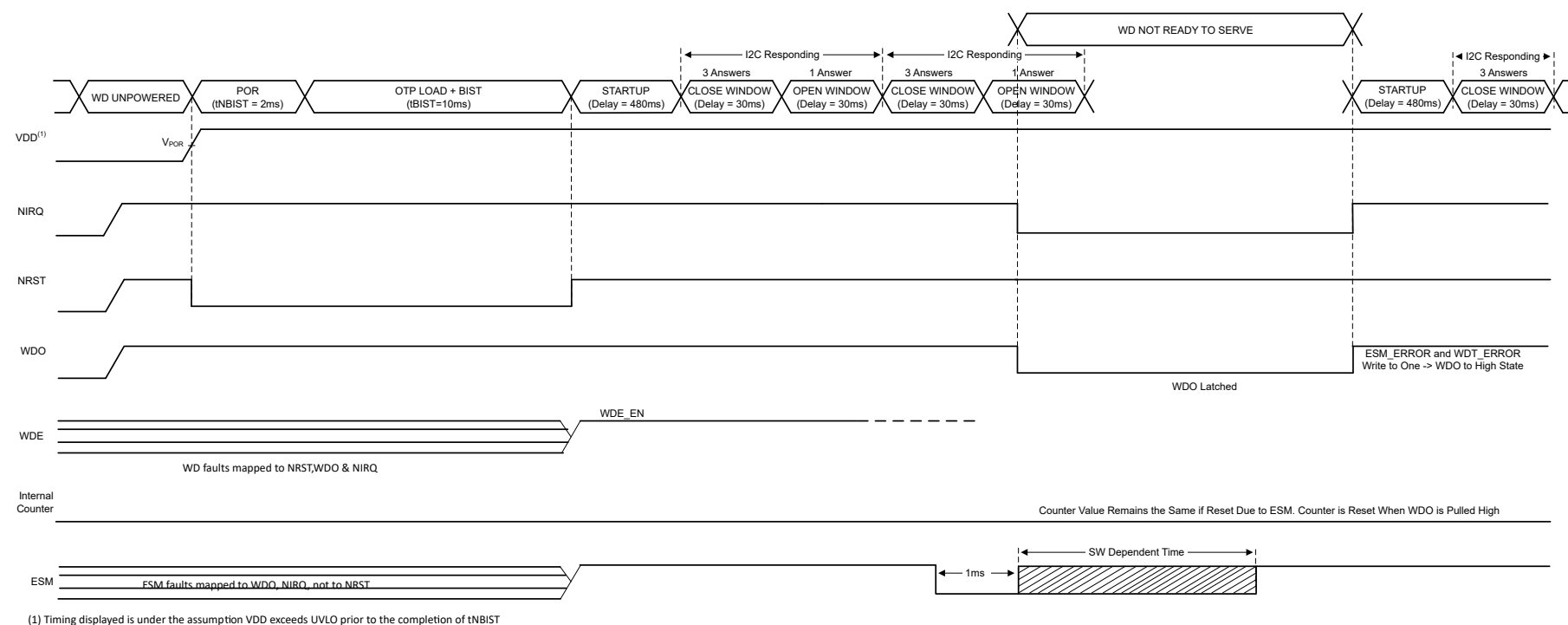
图 7-16. TPS389C03 ESM Error with No WD Faults
