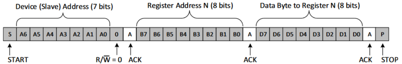
图 7-3. I 2 C write protocol
