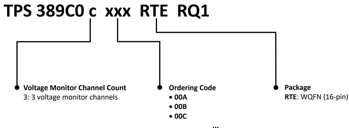
图 4-1. TPS389C03-Q1 Device Nomenclature
