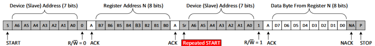
图 7-4. I 2 C read protocol
