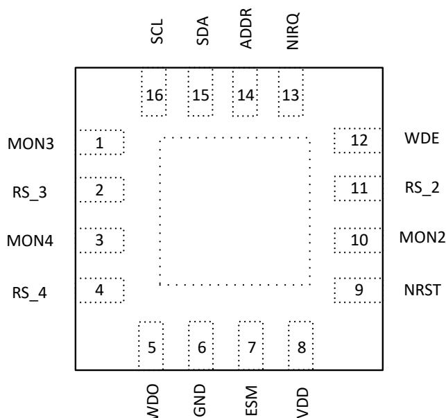
图 5-1. RTE Package 16-Pin WQFN TPS389C03-Q1 Top View
