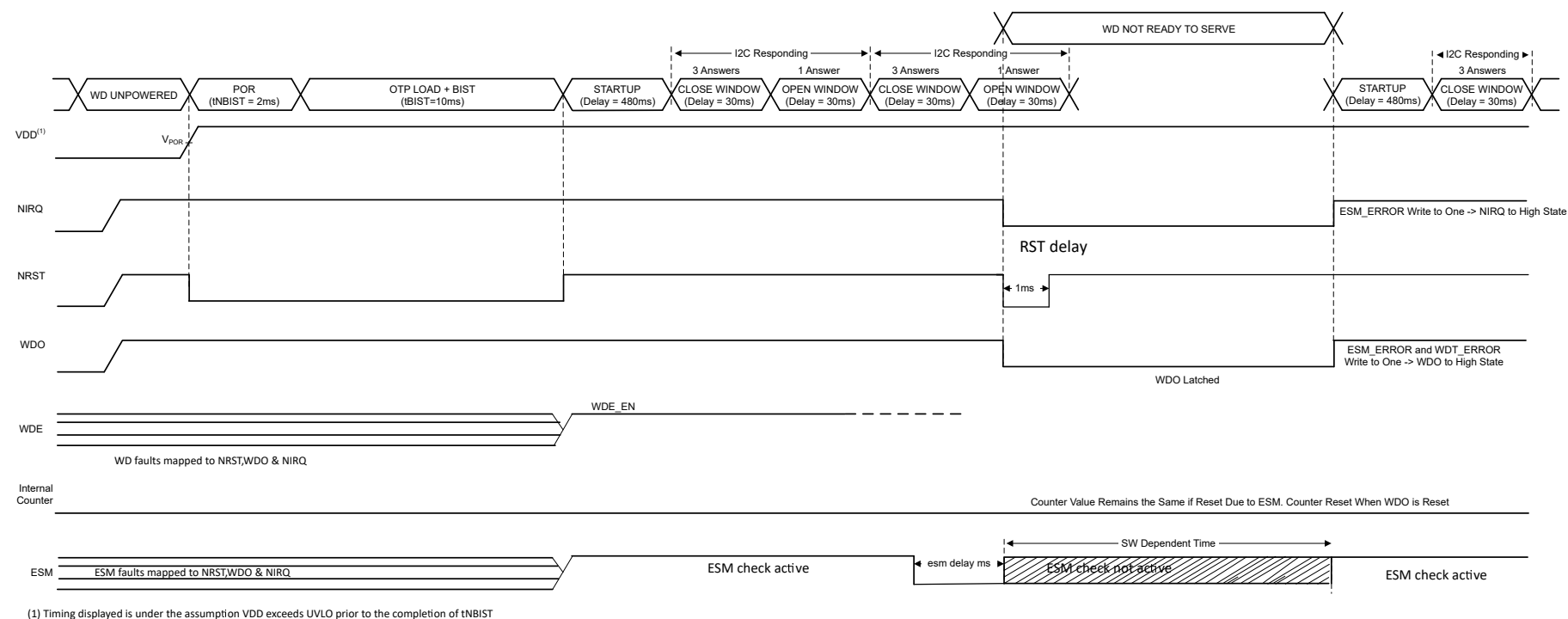
图 7-25. ESM Fault (WD Enabled)
