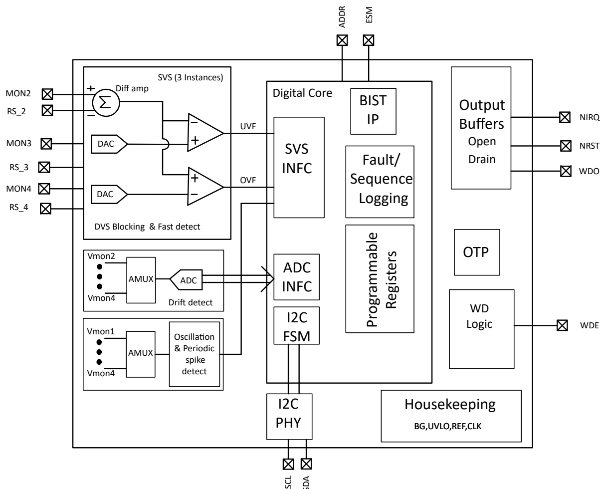
图 7-1. TPS389C03-Q1 Block Diagram
