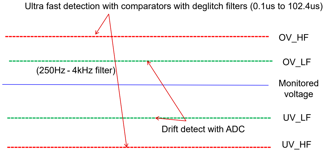
图 7-6. MON Channel State Diagram
