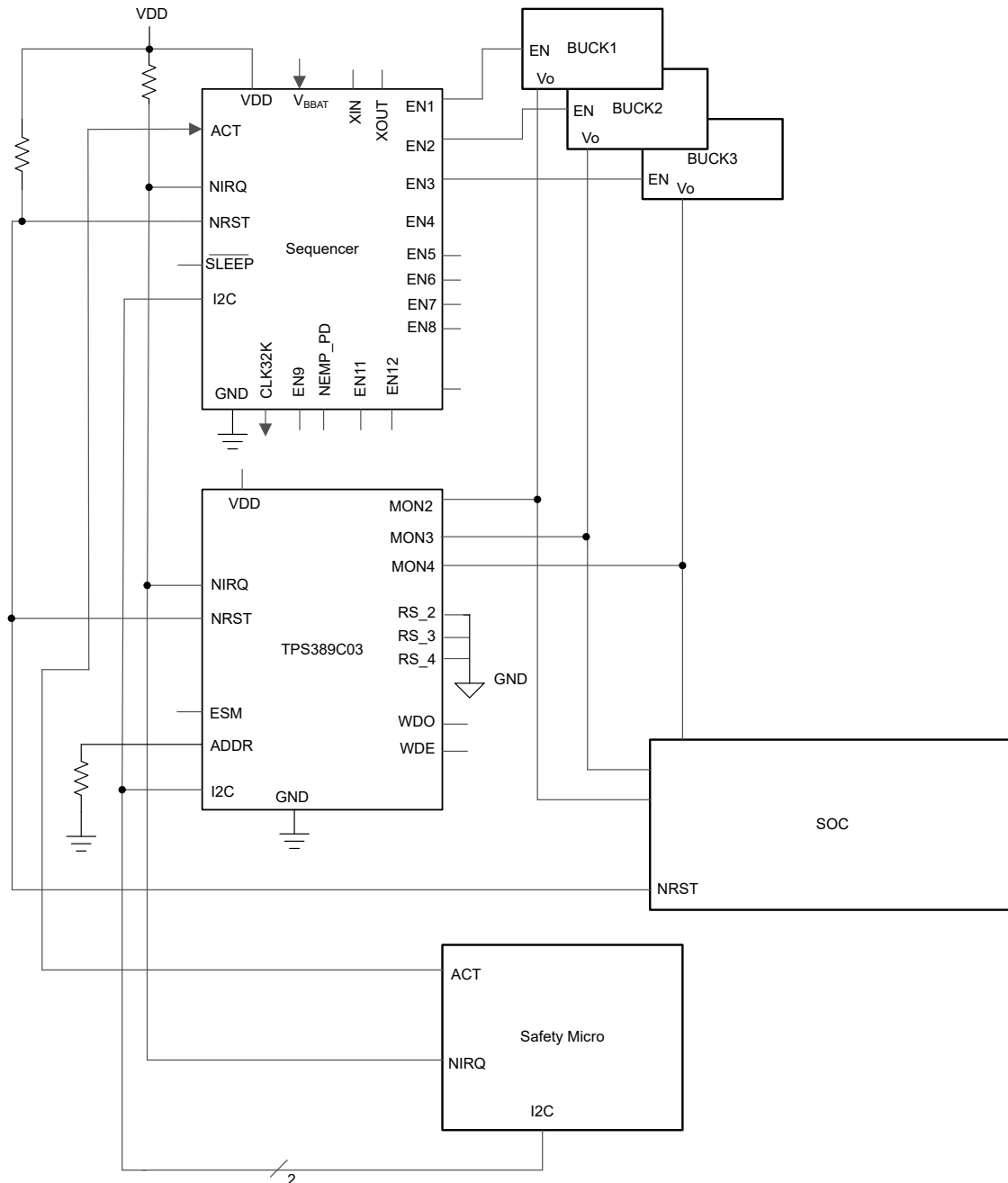
图 9-1. TPS389C03-Q1 Voltage Monitor Design Block Diagram
