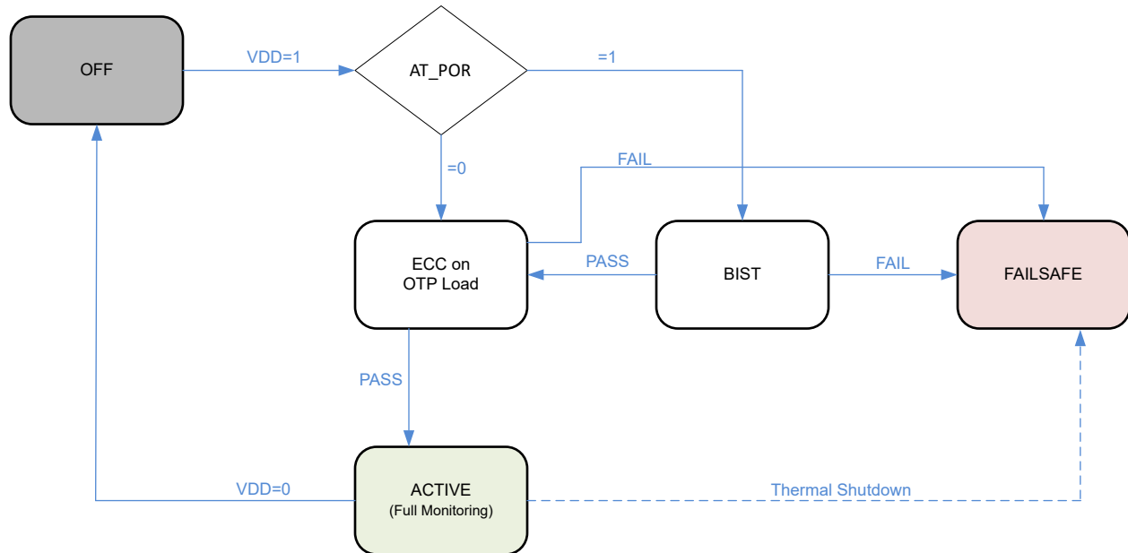
图 7-28. TPS389C03-Q1 State Diagram
