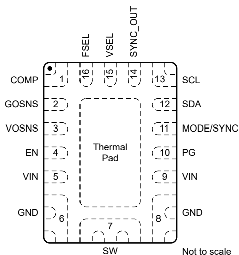
图 6-1. 16-Pin RXS VQFN Package (Top View)
