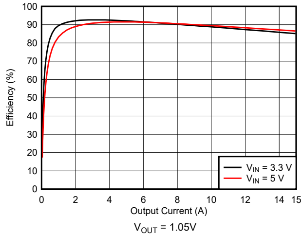
图 10-10. Efficiency
