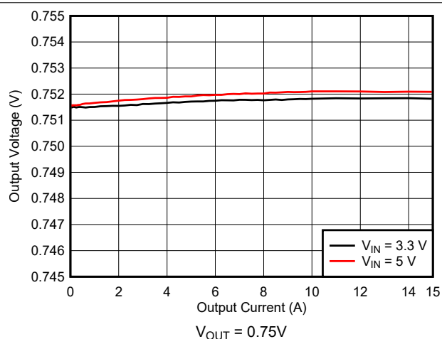
图 10-7. Load Regulation
