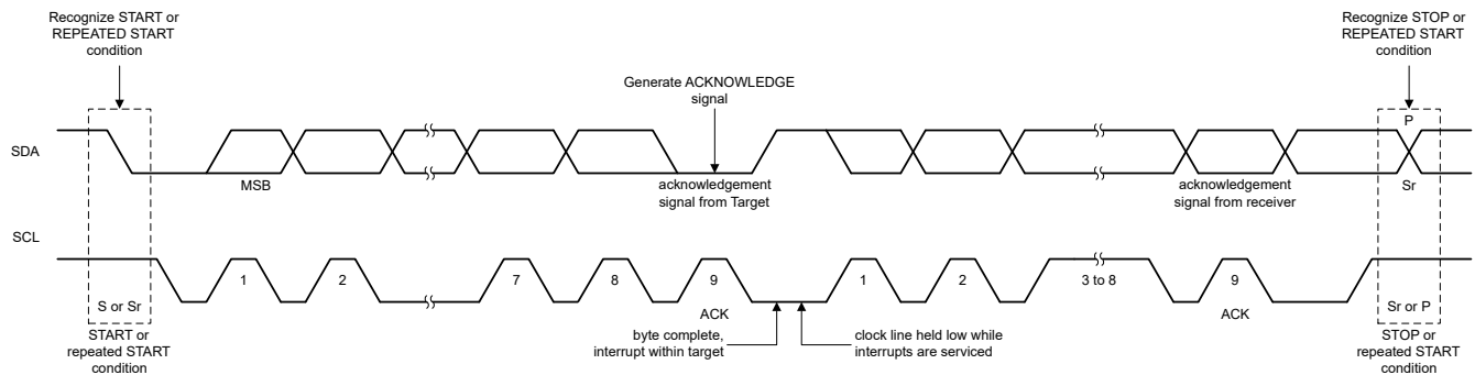
图 8-18. Bus Protocol
