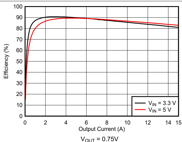
图 10-6. Efficiency
