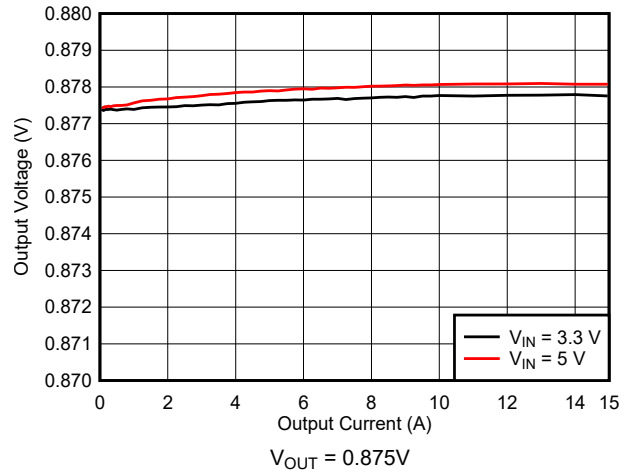
图 10-9. Load Regulation
