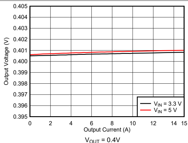
图 10-3. Load Regulation
