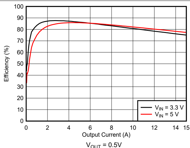
图 10-4. Efficiency
