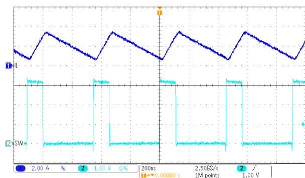
图 10-16. PWM-CCM Operation
