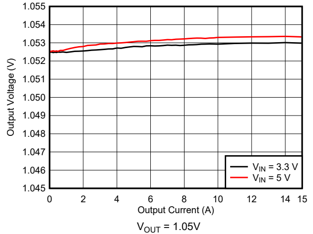
图 10-11. Load Regulation
