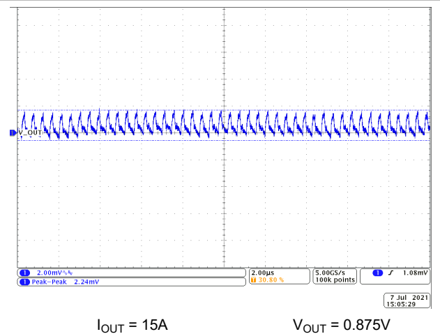
图 10-13. Output Voltage Ripple
