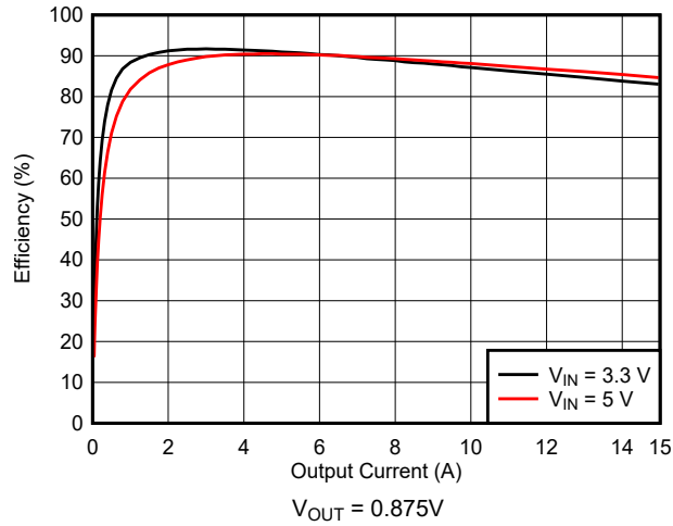
图 10-8. Efficiency
