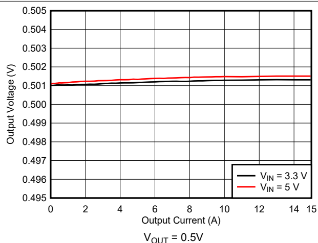
图 10-5. Load Regulation
