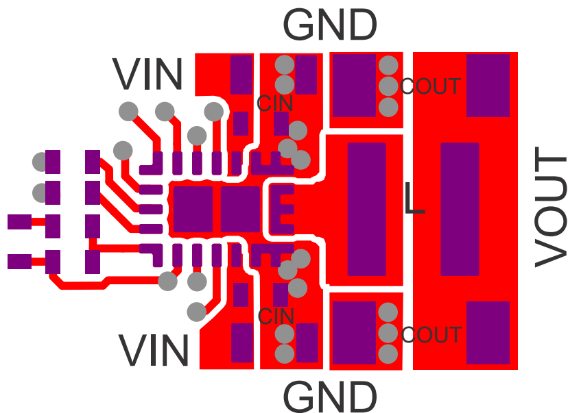
图 10-25. Layout Example
