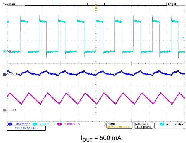
图 8-11. PWM Operation
