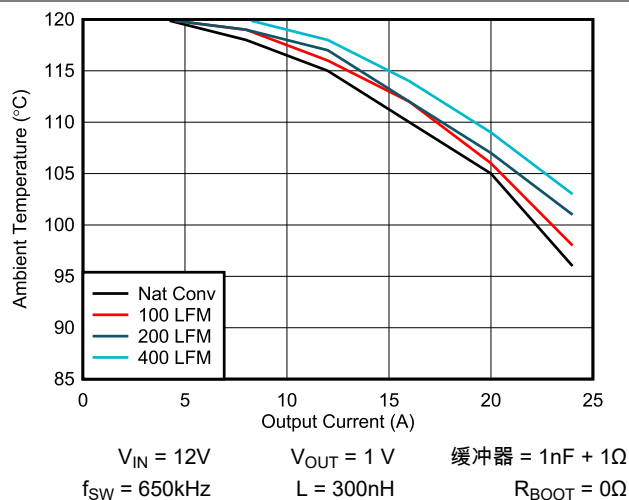
图 5-1. TPS546B24S 安全工作区
