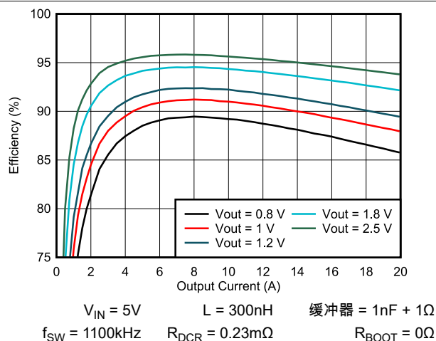
图 5-3. TPS546B24S 效率与输出电流间的关系
