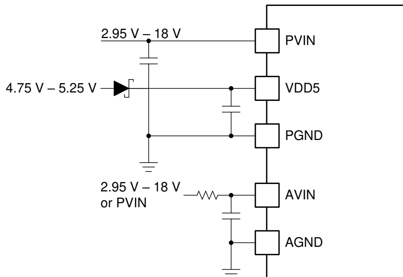
图 6-4. TPS546B24S 单独的 PVIN、AVIN 和 VDD5 连接
