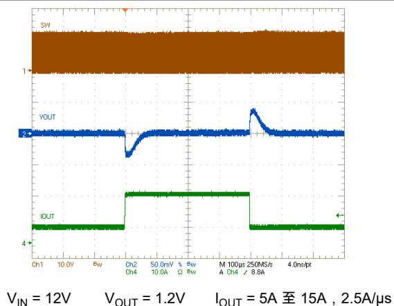
图 7-7. 负载瞬态响应
