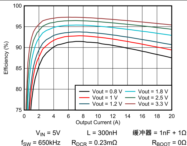
图 5-2. TPS546B24S 效率与输出电流间的关系
