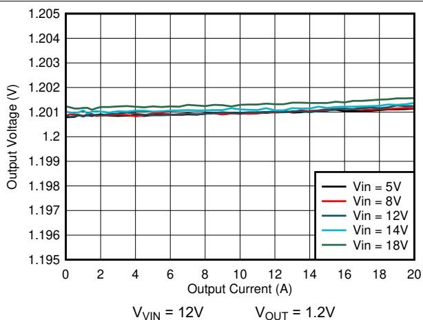
图 7-3. 负载调整率
