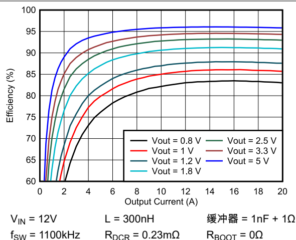
图 5-5. TPS546B24S 效率与输出电流间的关系
