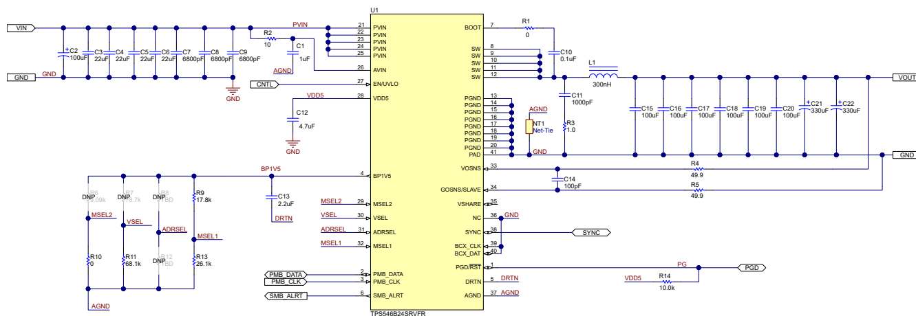
图 7-1. TPS546B24S 应用
