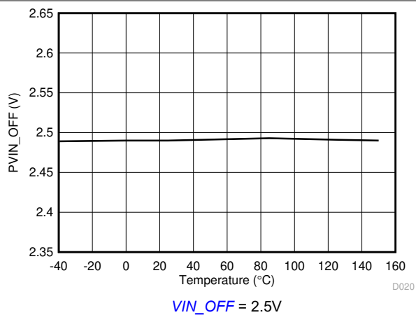
图 5-14. 关断电压与结温间的关系
