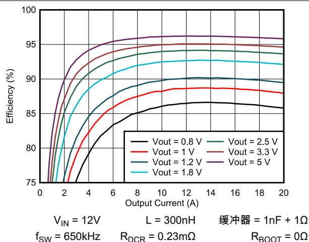
图 5-4. TPS546B24S 效率与输出电流间的关系
