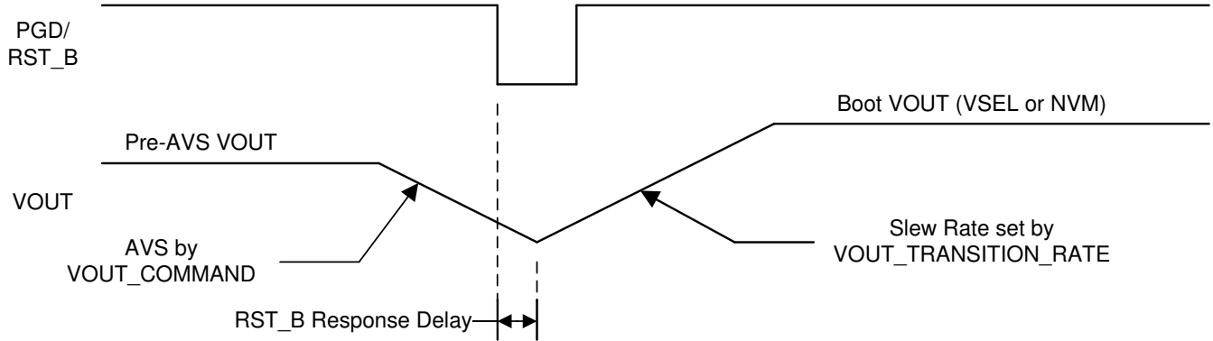
图 6-7. TPS546B24S 输出电压复位
