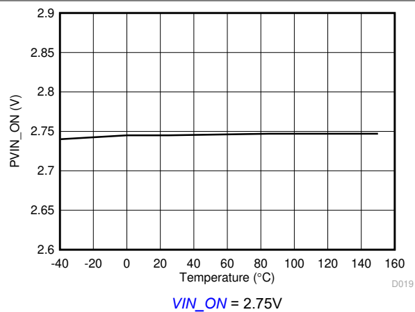
图 5-13. 导通电压与结温间的关系
