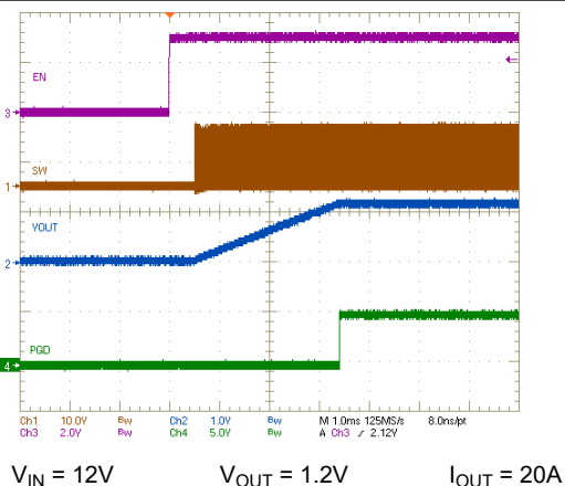
图 7-5. 从 EN/UVLO 启动
