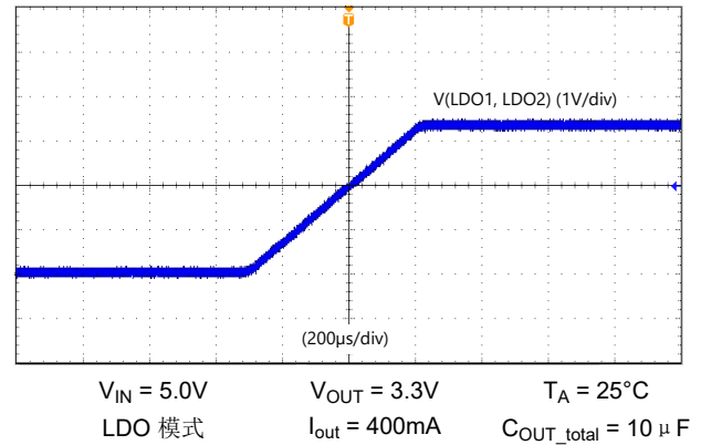
图 7-5. LDO1 斜坡
