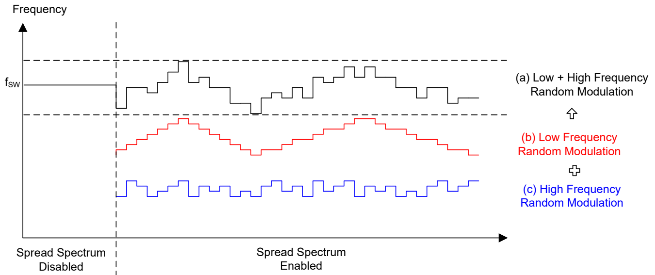
图 6-4. 双随机展频
