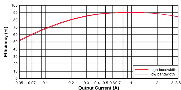
图 5-2. BUCK1 效率
