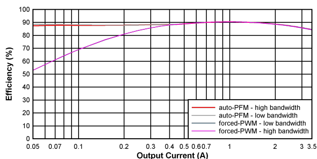
图 5-1. BUCK1 效率
