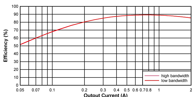
图 5-1. BUCK1 效率
