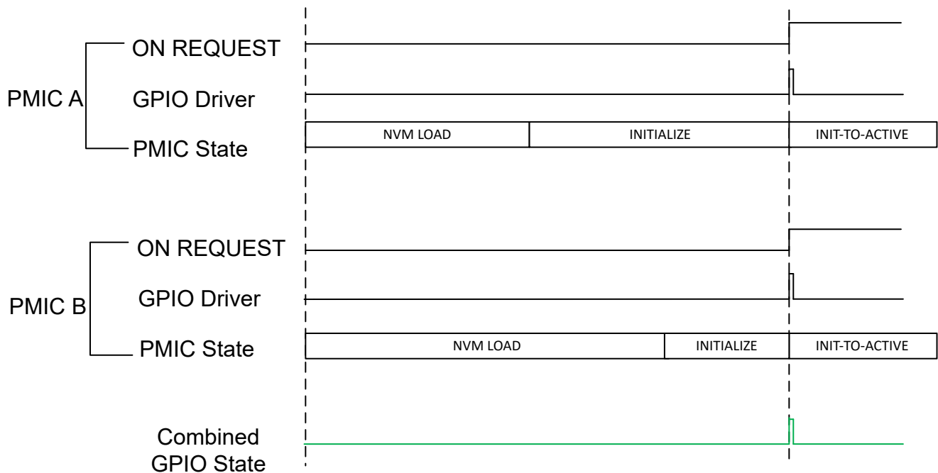
图 6-13. 上电前同步
