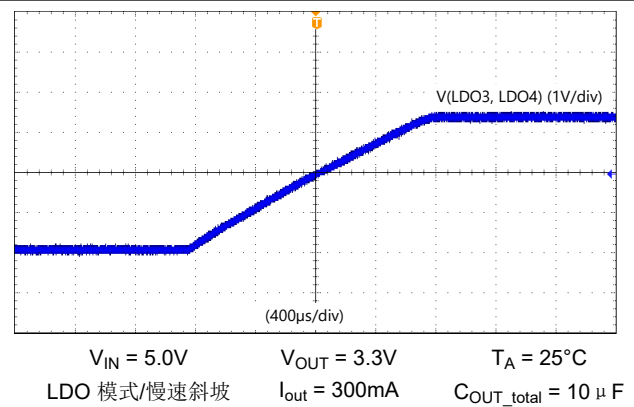
图 7-7. LDO 慢速斜坡
