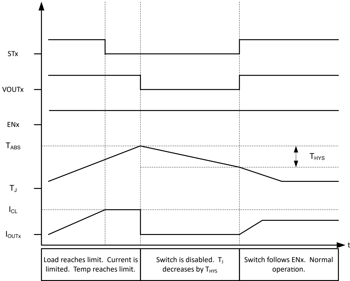
图 8-9. Thermal Shutdown - Auto-retry Behavior
