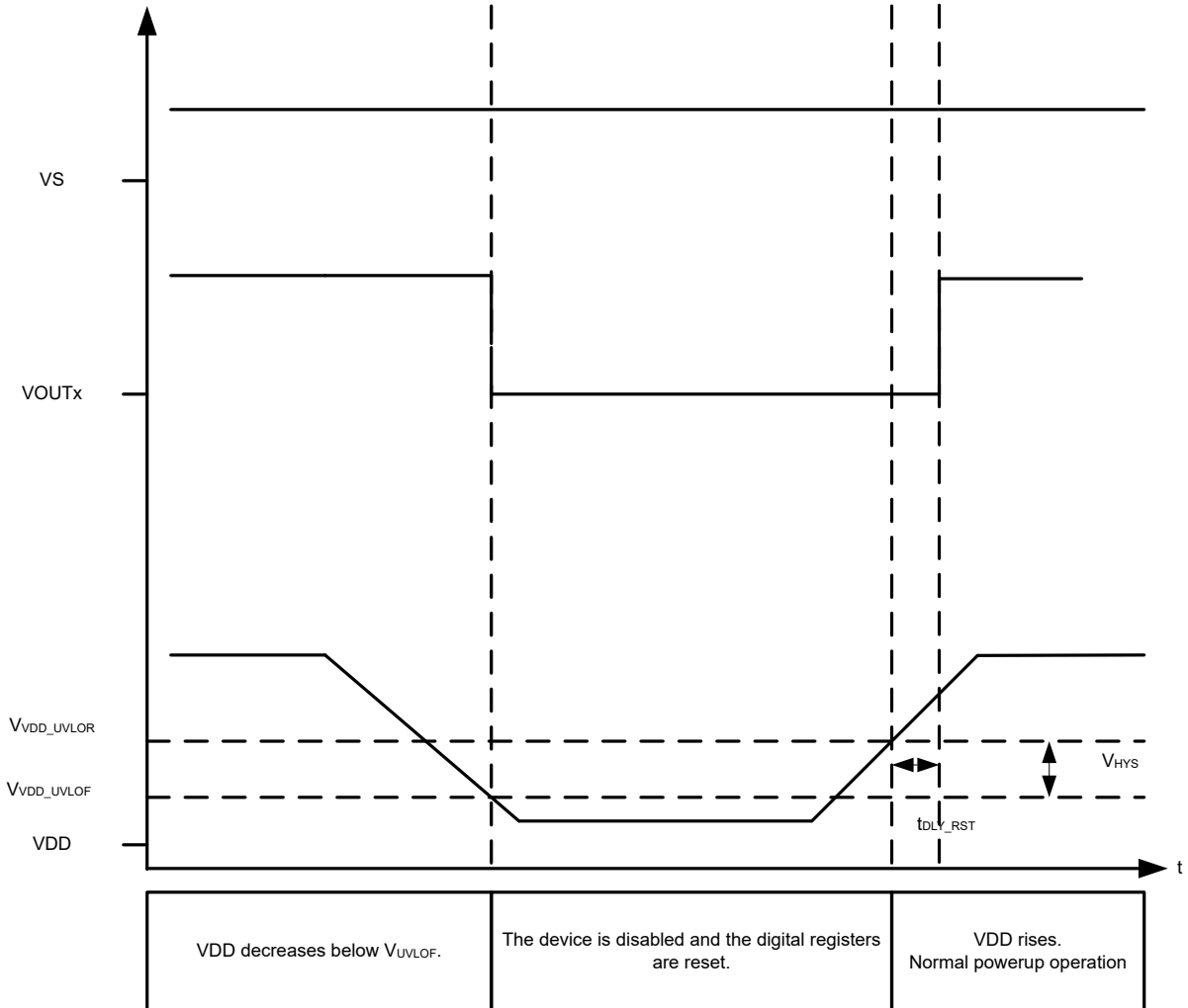
图 8-14. VDD UVLO
