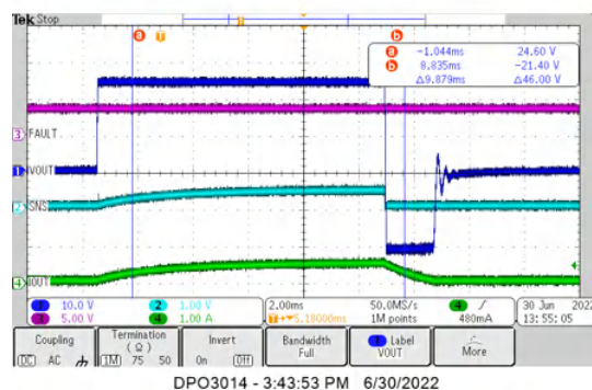
图 8-12. TPS274C65 Inductive Discharge (100 mH + 48 \Omega )
