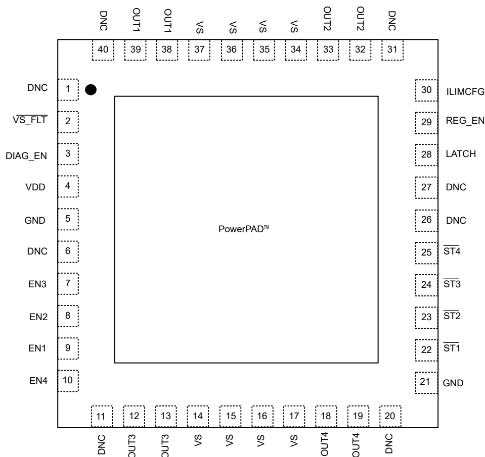
图 5-1. RHA Package, 40-Pin VQFN (Top View)
