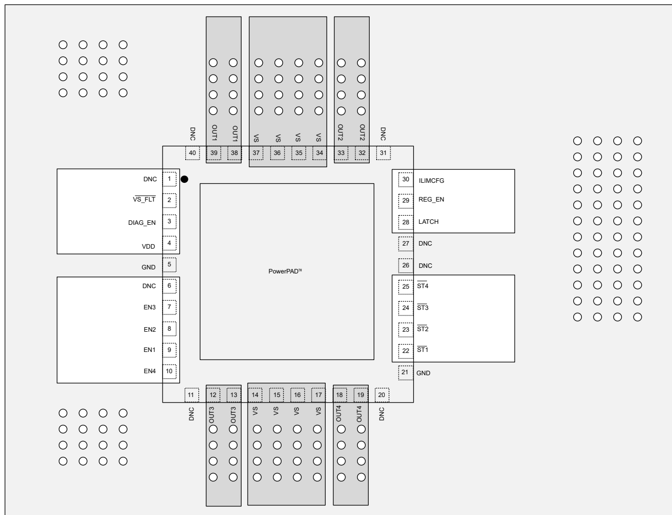
图 9-4. TPS274C65CP Layout Example
