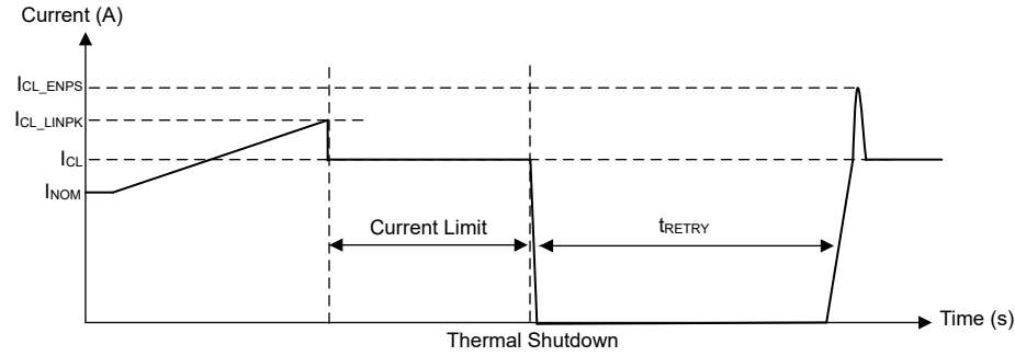
图 8-7. Soft Short-Circuit Behavior
