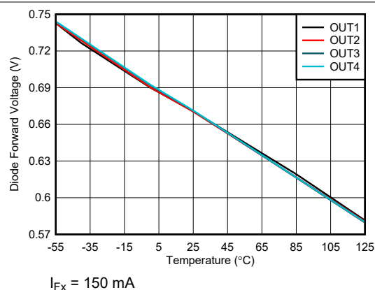
图 6-6. Body-Diode Forward Voltage
