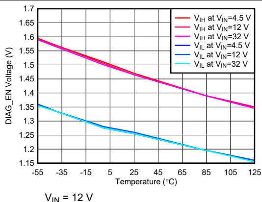
图 6-3. DIAG_EN Voltage Threshold
