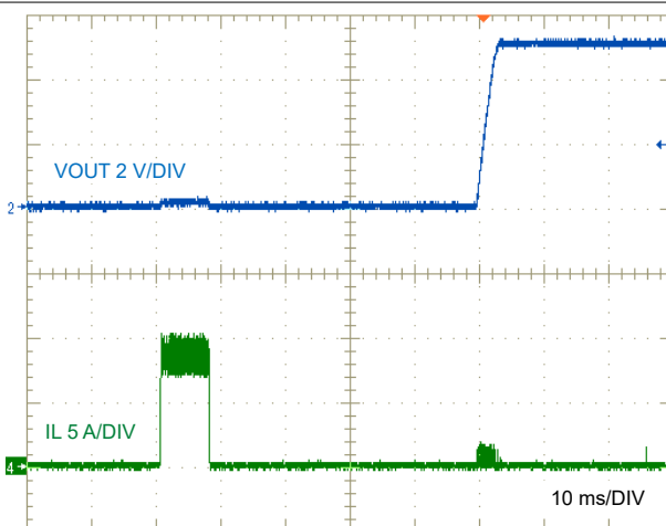
图 9-9. LM64460-Q1 Short-Circuit Recovery to No Load
