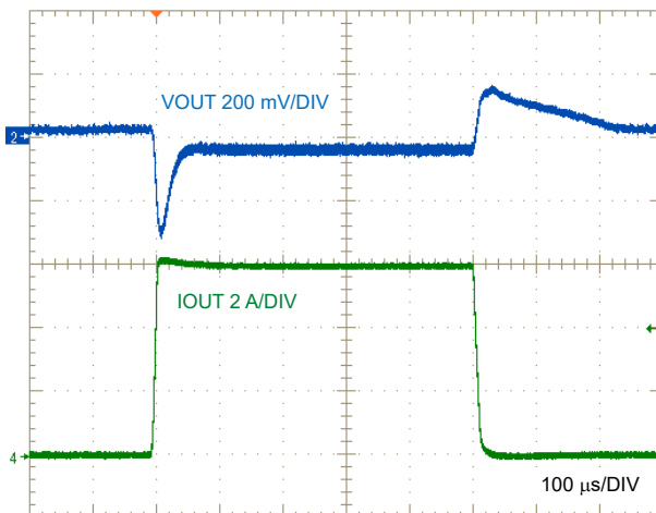
图 9-7. LM64460-Q1 Load Transient, I_{OUT} = 0 \text{ A to } 6 \text{ A}
