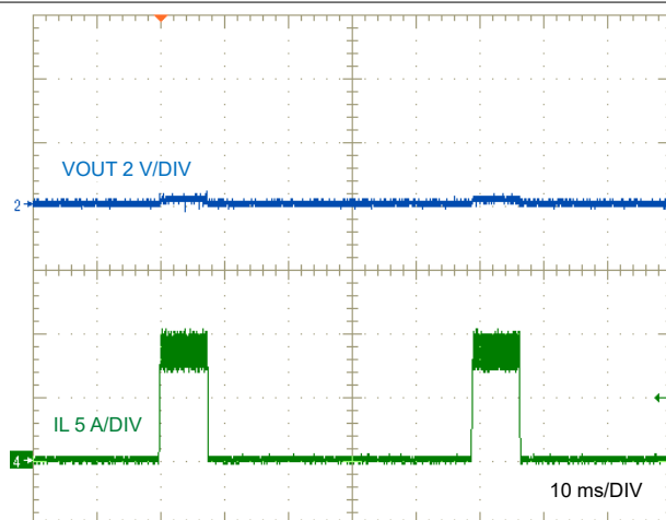
图 9-8. LM64460-Q1 Short-Circuit Hiccup
