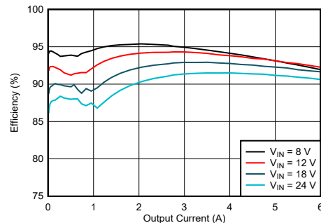
效率图， V_{OUT} = 5V ， f_{SW} = 2.1MHz
