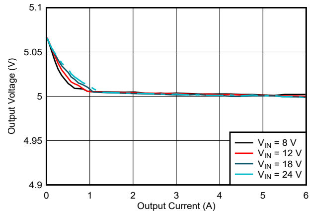
图 9-3. LM64460-Q1 Load and Line Regulation
