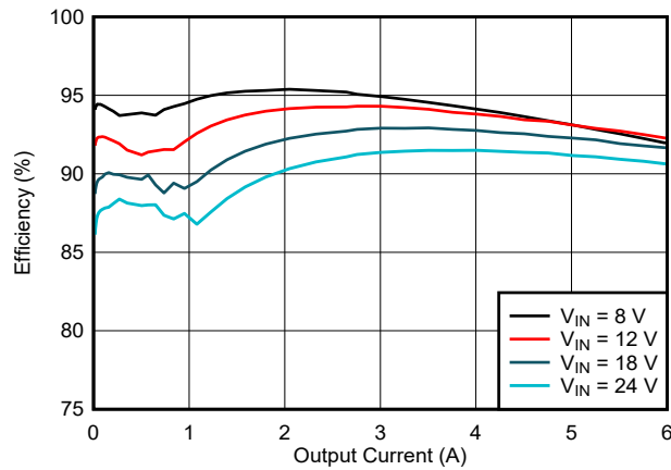
图 9-2. LM64460-Q1 Efficiency
