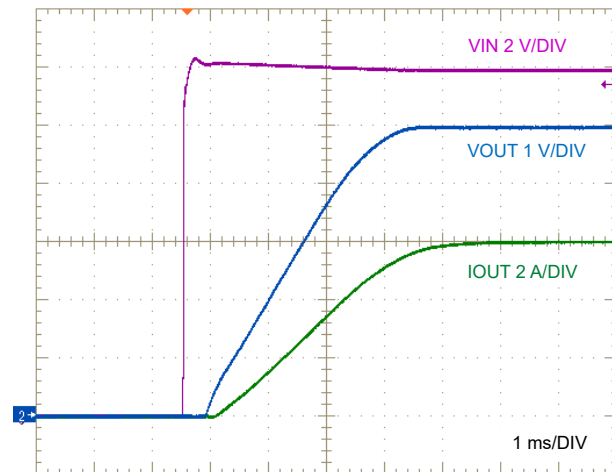
图 9-4. LM64460-Q1 Start-Up, 6-A Resistive Load
