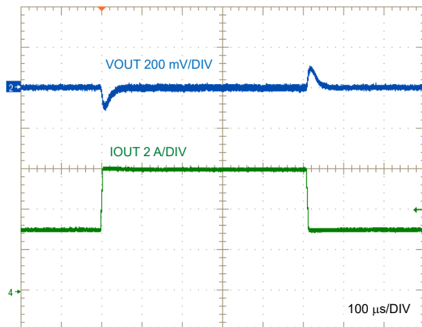
图 9-6. LM64460-Q1 Load Transient, I_{OUT} = 3 \text{ A to } 6 \text{ A}
