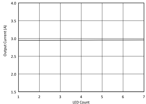
图 7-2. 输出电流与 LED 计数间的关系
