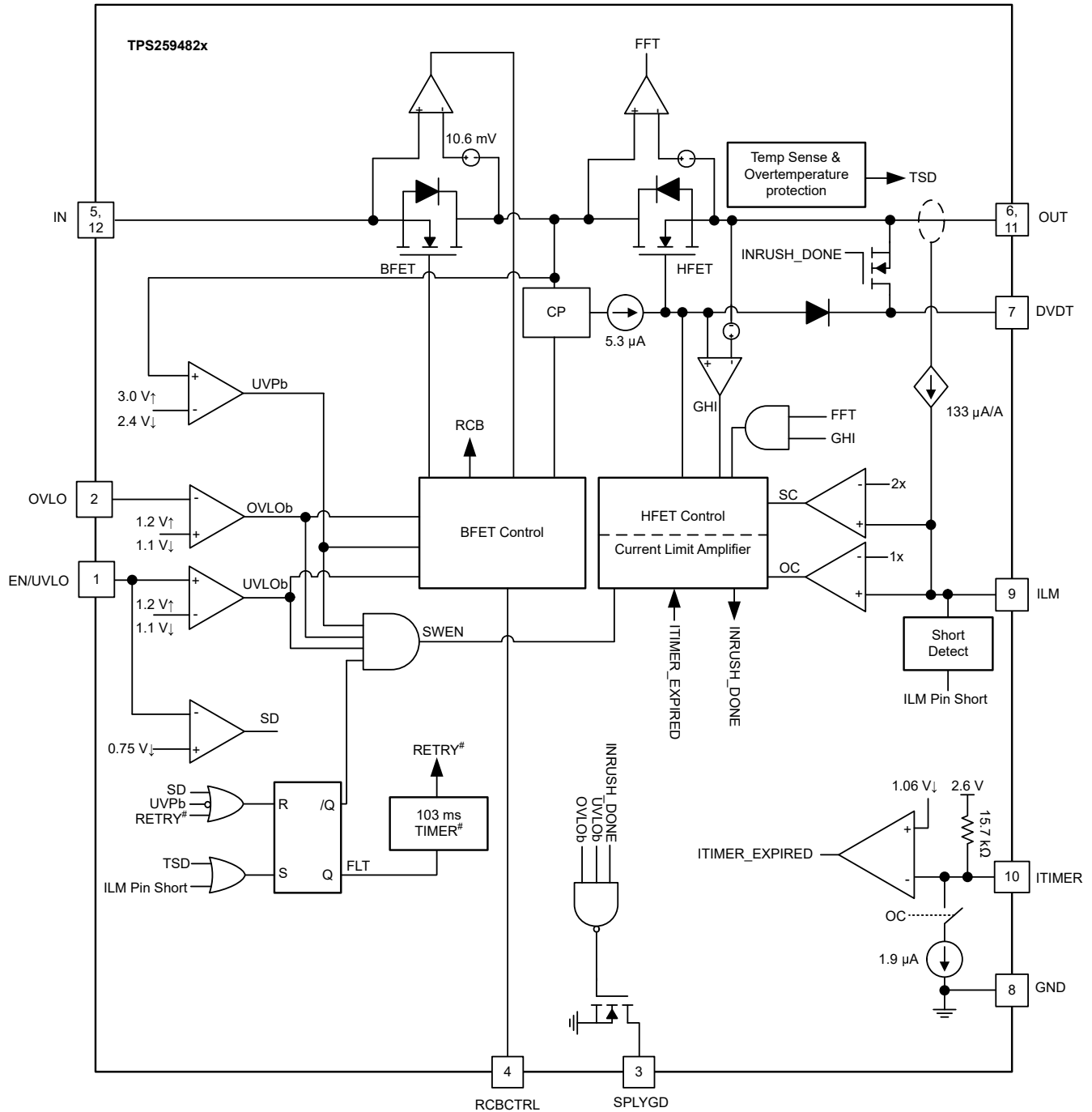
图 8-3. TPS259482x Block Diagram
