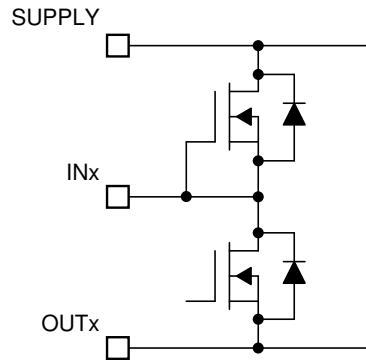
图 7-14. IN Pin
