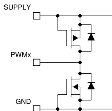
图 7-9. PWM Pin
