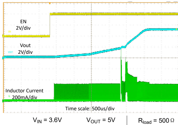
图 8-17. 由 EN 启动
