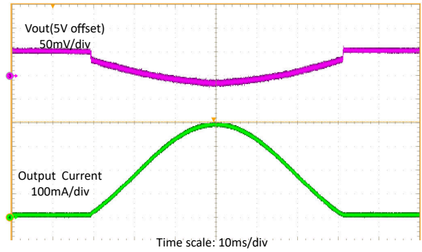
图 8-9. 负载扫描
