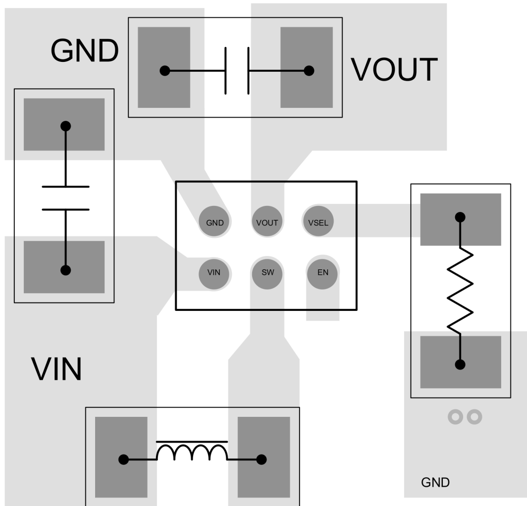
图 8-23. 布局示例 - YBH
