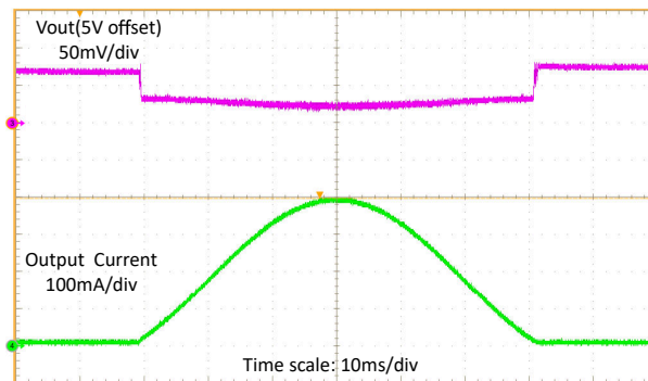
图 8-20. 负载扫描
