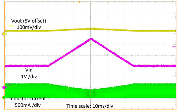
图 8-11. 线路扫描
