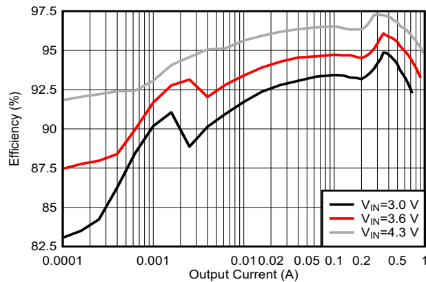
图 6-3. 不同输入电压在正常模式下的 3.3V VOUT 效率
