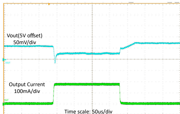
图 8-19. 负载瞬态
