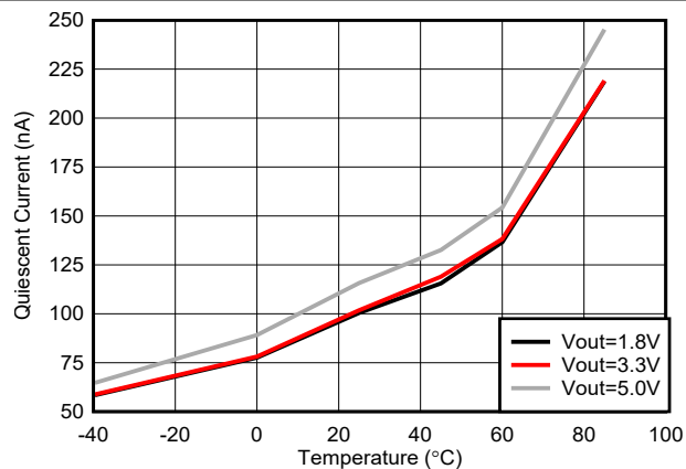
图 6-8. 流入 VOUT 的静态电流与温度间的关系
