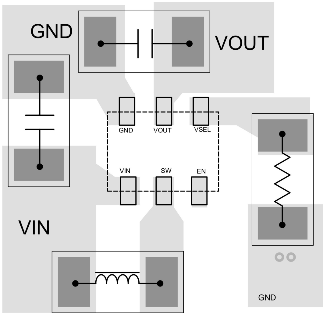
图 8-24. 布局示例 - DRL
