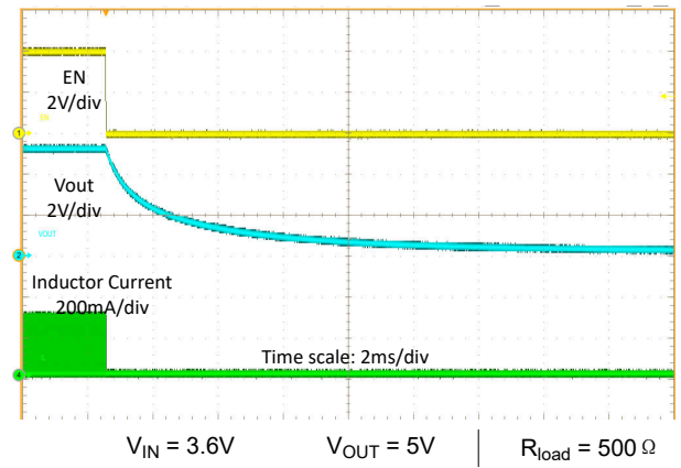
图 8-18. 由 EN 关断
