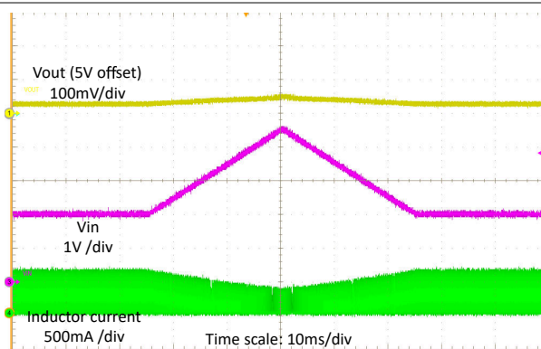
图 8-22. 线路扫描
