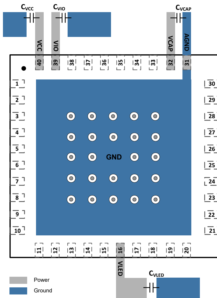
图 8-10. LP5860T 布局示例
