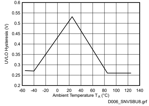
图 6-4. V_{CC} UVLO 迟滞
