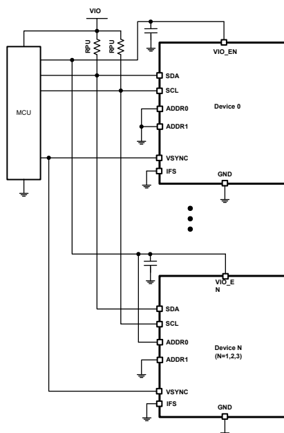
图 7-16. I 2 C 多器件连接
