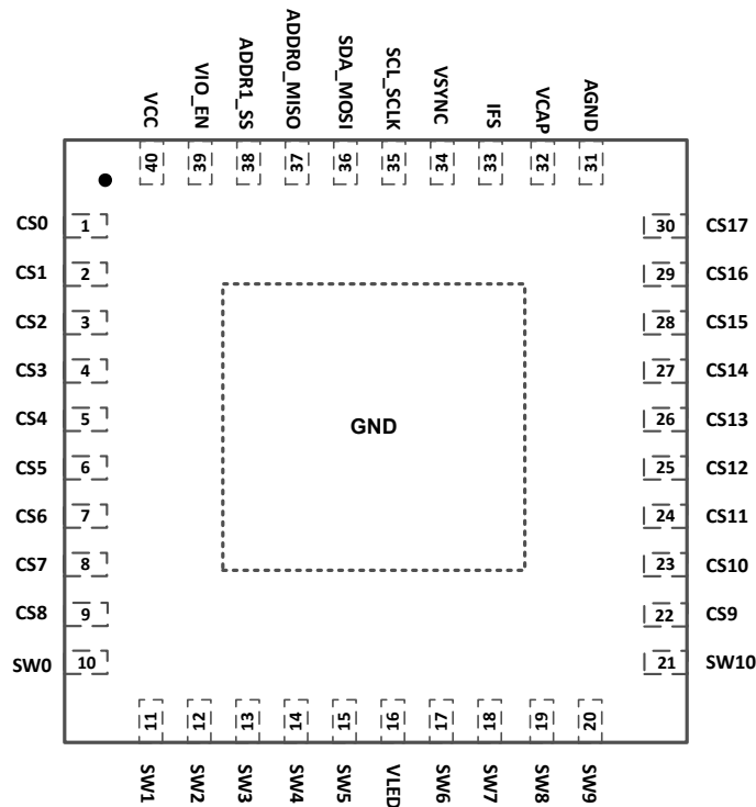
图 5-1. LP5860T RKP 封装 40 引脚 VQFN (带外露散热焊盘) 顶视图
