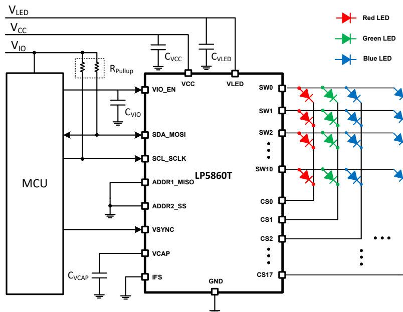
图 8-1. 典型应用 — LP5860T 驱动 66 个 RGB LED (198 个 LED 点阵)
