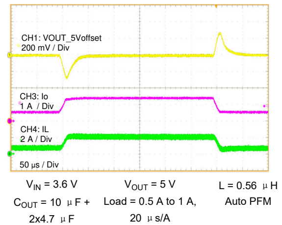
图 9-7. Load Transient
