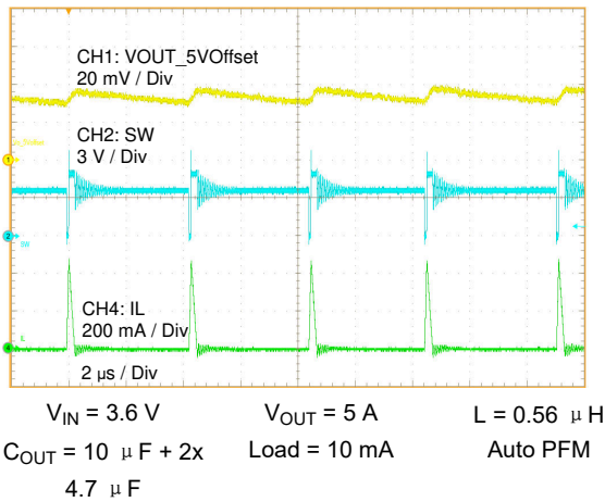
图 9-2. Steady 10 mA
