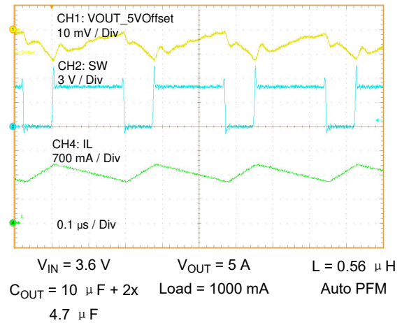
图 9-3. Steady 1000 mA
