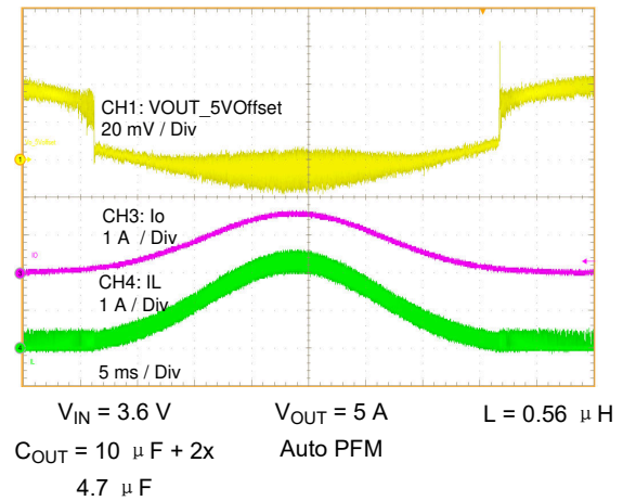
图 9-5. Load Sweep
