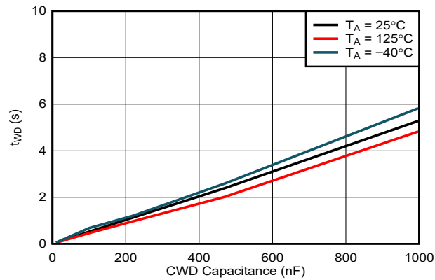
图 7-4. t_{WD} 与电容间的关系
