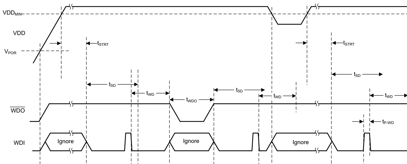
图 7-1. 功能时序图
