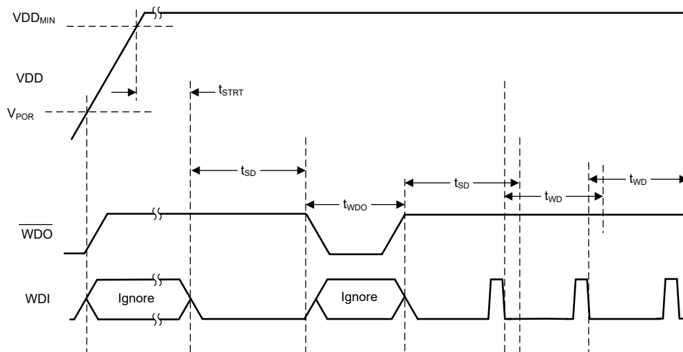
图 8-6. t_{SD} 帧行为
