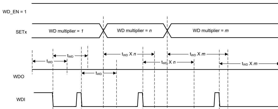
图 8-7. 具有 SETx 引脚状态的看门狗行为
