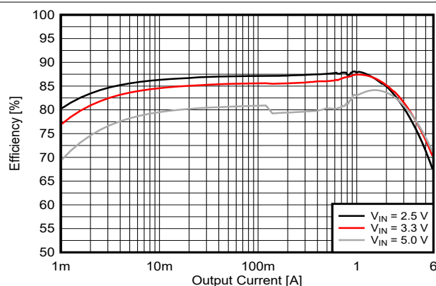
图 9-2. 0.6V 输出效率 (TPS62A06)
