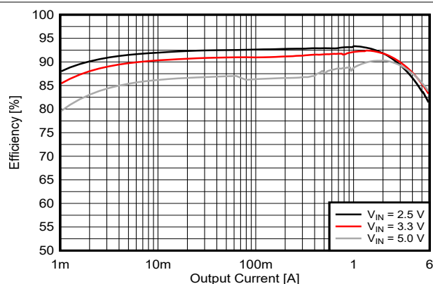
图 9-3. 1.2V 输出效率 (TPS62A06)
