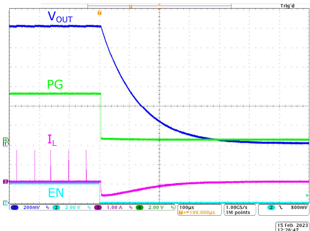
图 9-9. 在无负载条件下关断 (TPS62A06)
