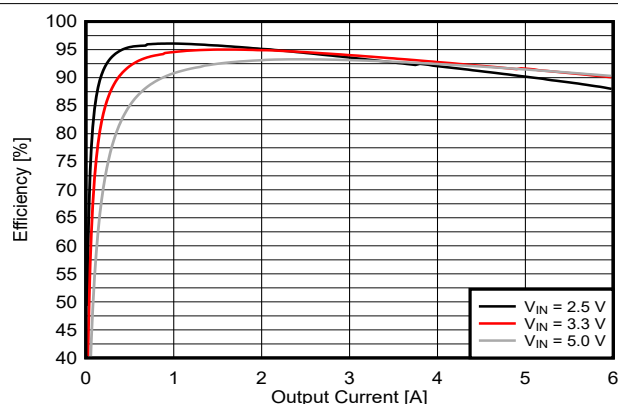
图 9-5. 1.8V 输出效率 (TPS62A06A)
