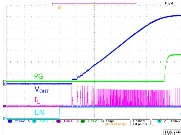
图 9-8. 在无负载条件下启动 (TPS62A06)
