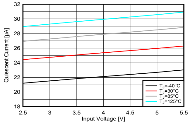
图 7-1. 静态电流与输入电压间的关系
