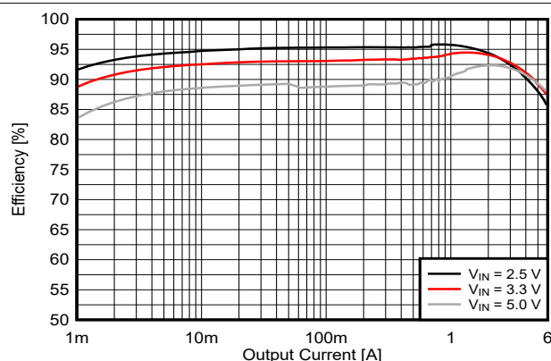
图 9-4. 1.8V 输出效率 (TPS62A06)
