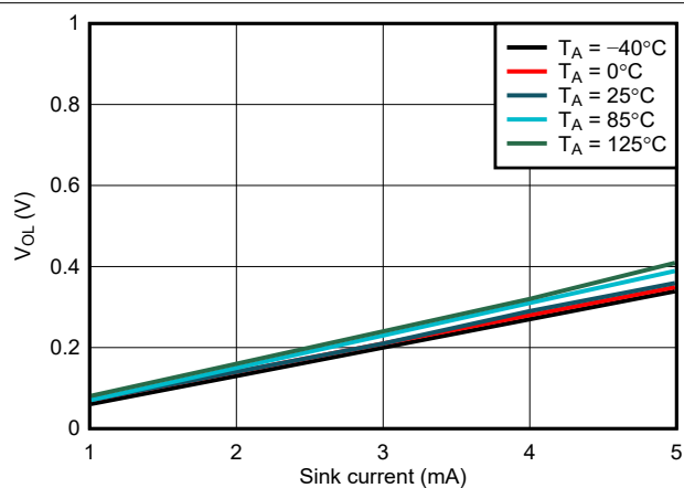
图 7-6. WDO V_{OL} 与 I_{sink} 间的关系, V_{DD} = 1.5\text{V}
