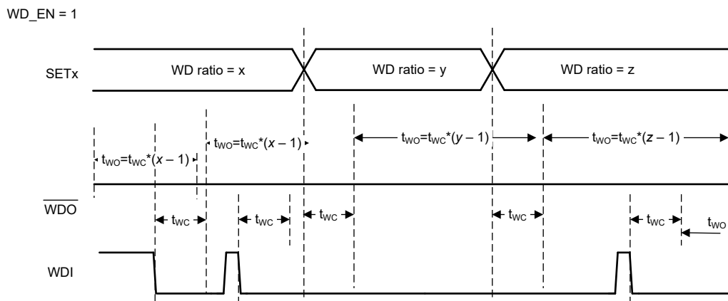
图 8-7. 具有 SETx 引脚状态的看门狗行为
