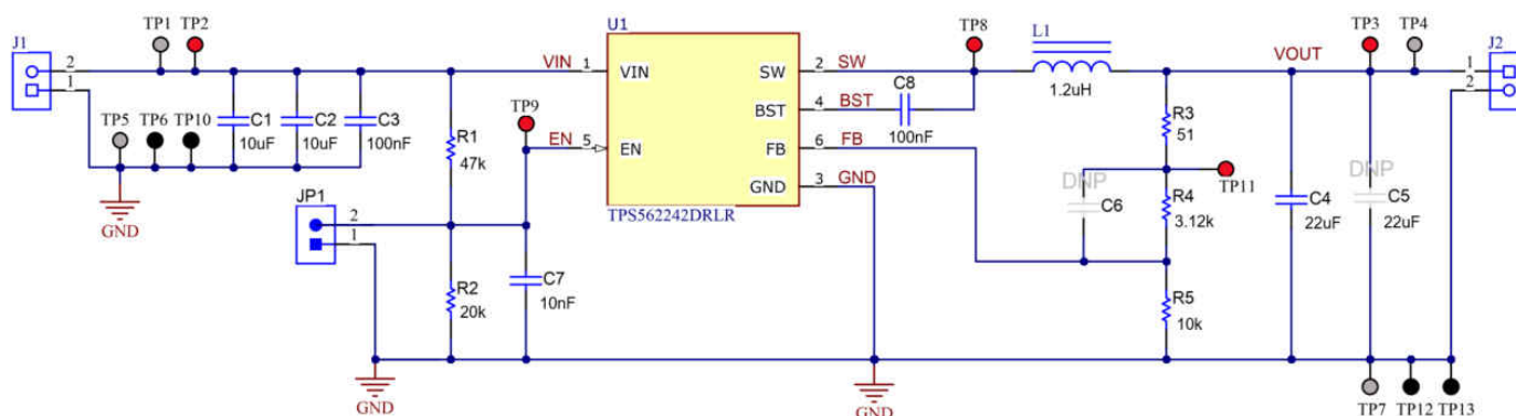
图 8-1. Schematic
