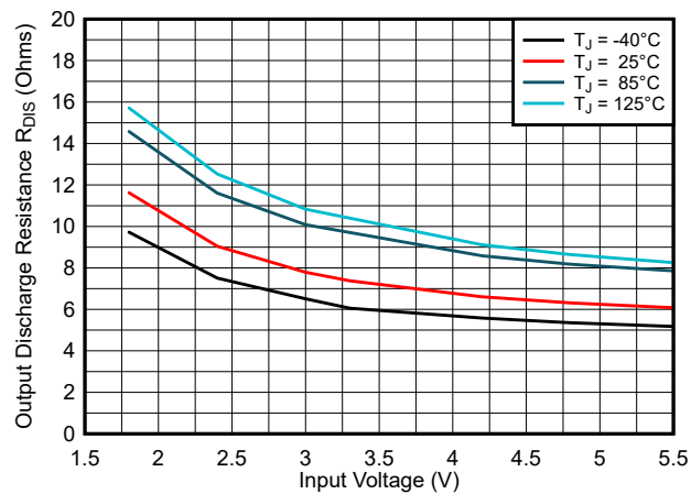
图 6-5. VOS Discharge Switch Drain Source Resistance R_{DIS}
