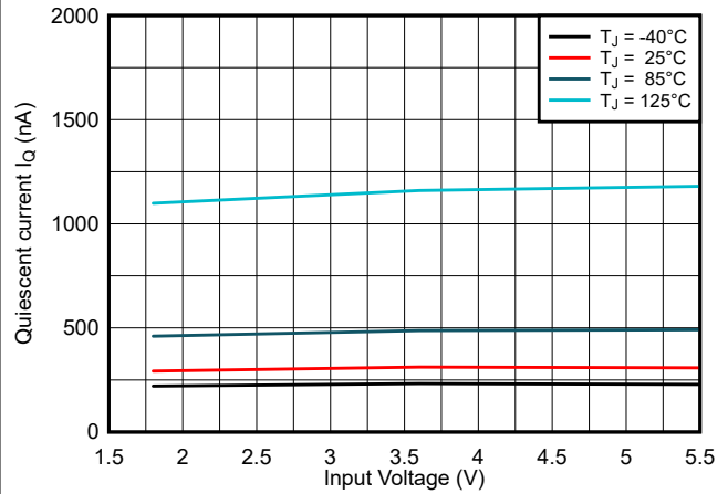
图 6-2. Quiescent Current I_Q
