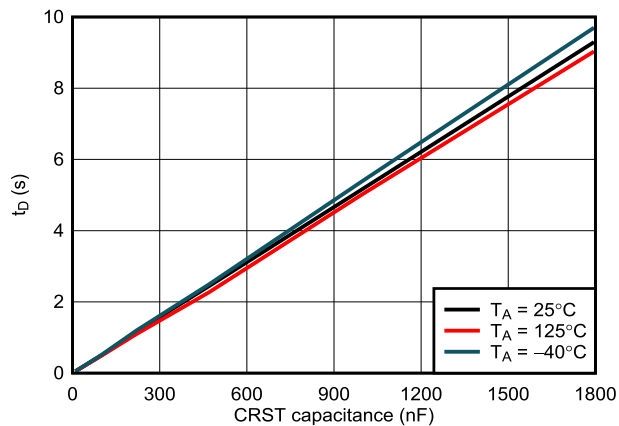
图 7-9. t_D vs Capacitance
