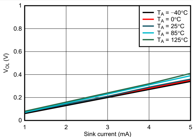
图 7-11. WDO V_{OL} vs I_{sink} , V_{DD} = 1.5\text{ V}
