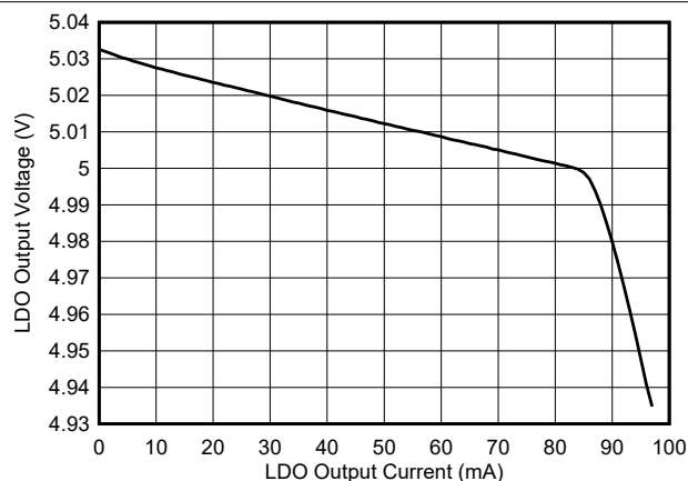
图 5-9. LDO Output Load Regulation
