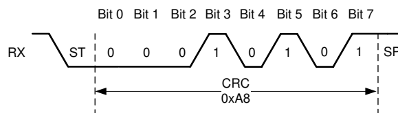
图 6-15. CRC Byte
