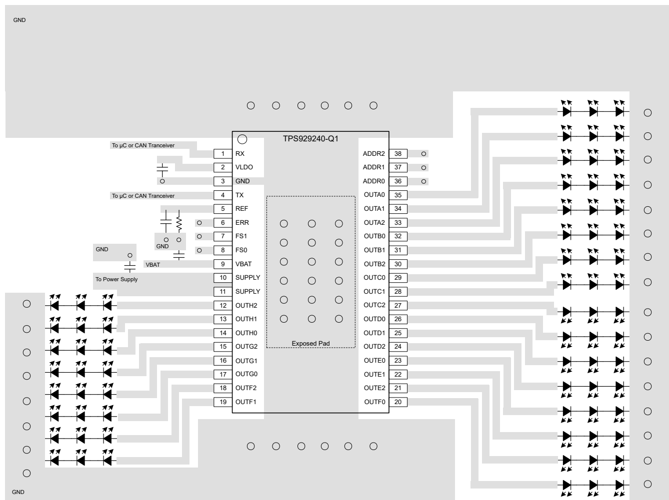
图 7-5. TPS929240-Q1 Layout
