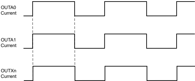
图 6-3. PWM Dimming Mode
