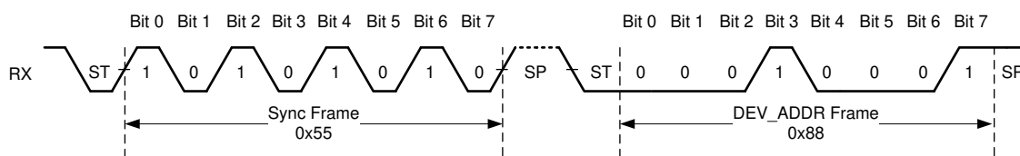
图 6-13. Synchronization Byte
