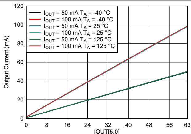
图 5-7. Output DC Current vs IOUT[5:0]
