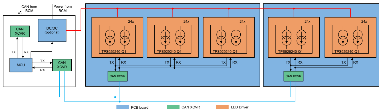
图 7-1. System Block Diagram
