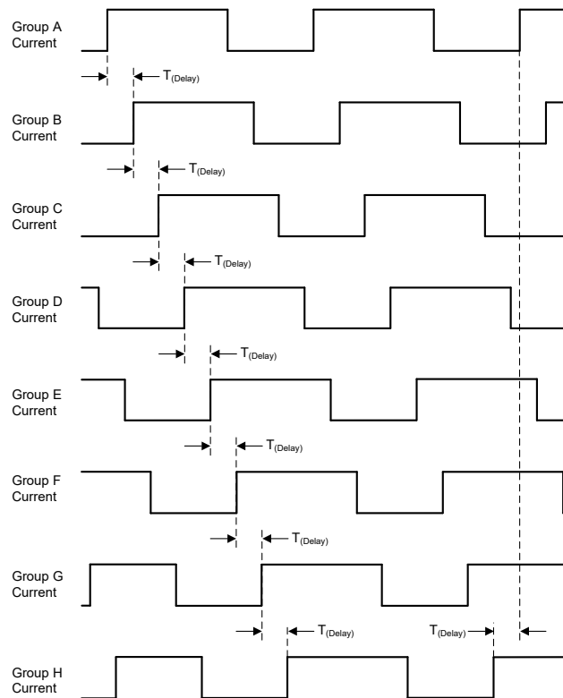
图 6-4. Phase Shift Dimming Mode
