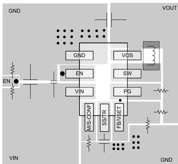
图 9-69. Layout
