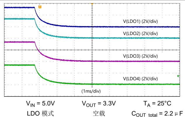
图 8-9. LDO 放电
