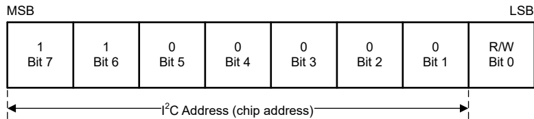
图 7-7. 示例器件地址
