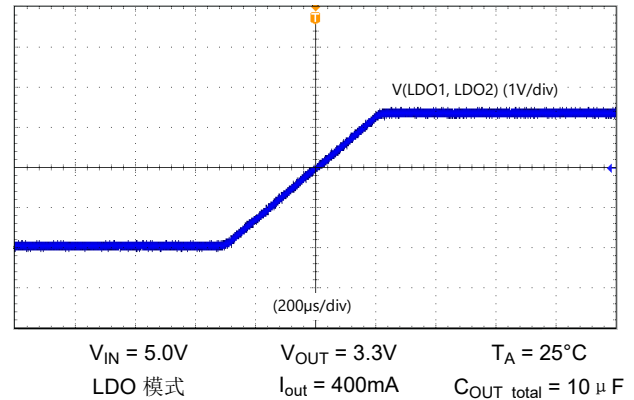
图 8-5. LDO1、LDO2 斜坡
