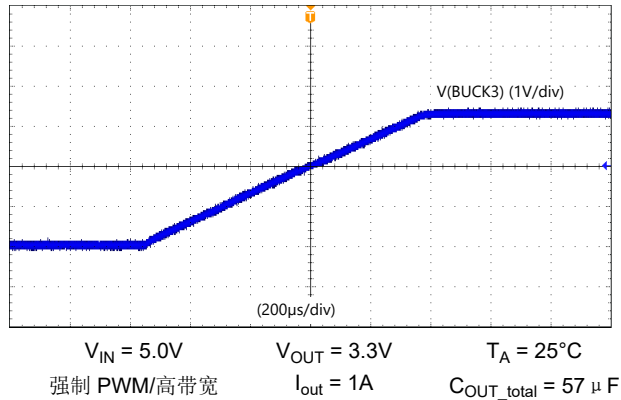
图 8-4. Buck3 斜坡
