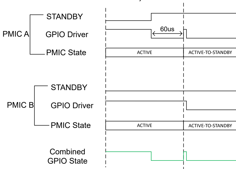
图 7-14. 转换到待机/OFF 请求/冷复位前同步
