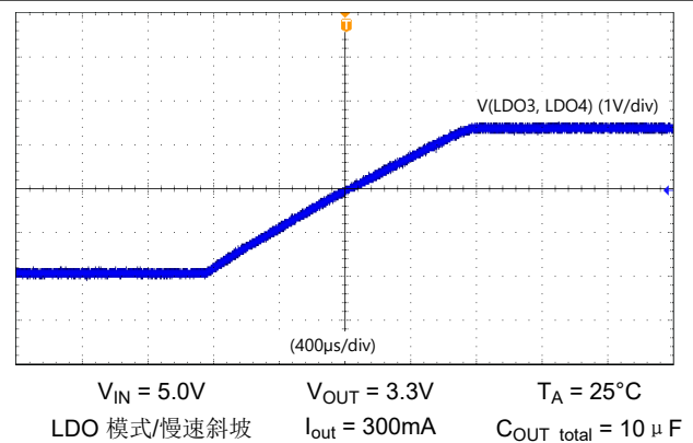
图 8-7. LDO3、LDO4 慢速斜坡
