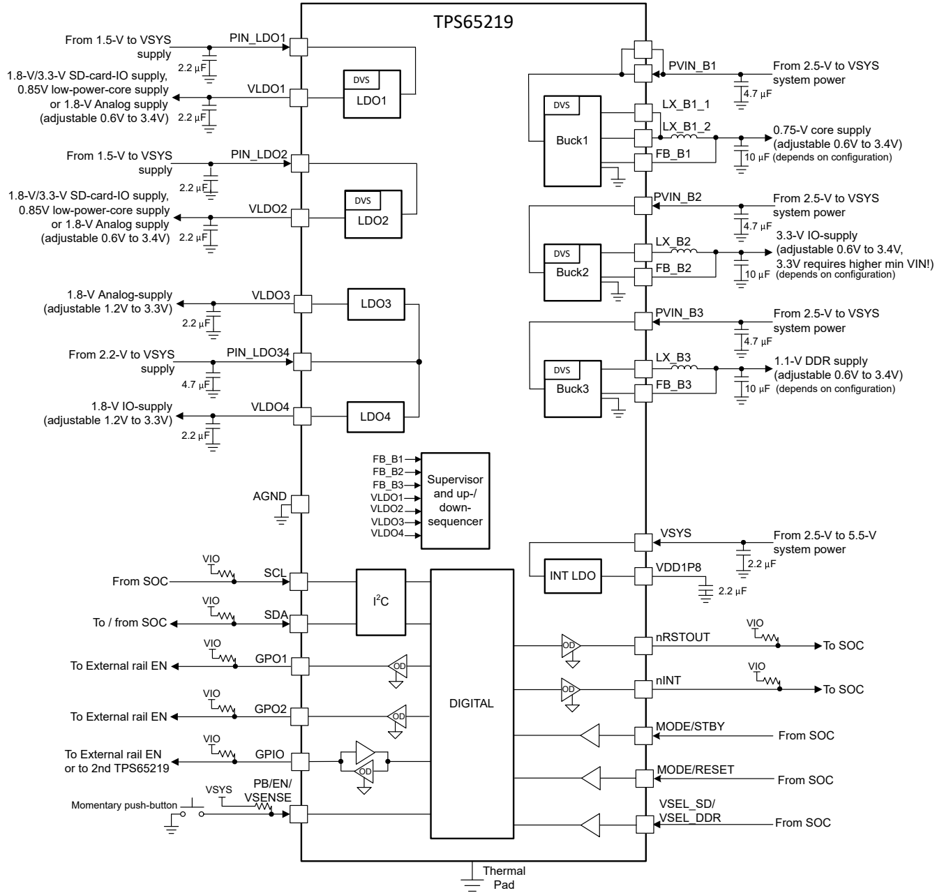
图 7-1. 功能方框图
