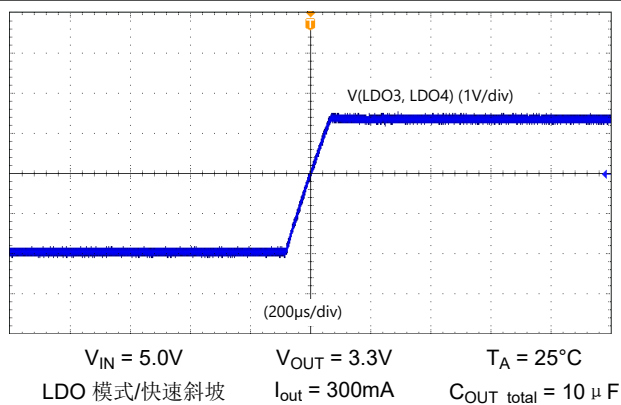
图 8-6. LDO3、LDO4 快速斜坡
