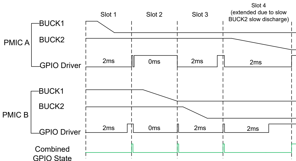
图 7-15. 断电序列期间的同步
