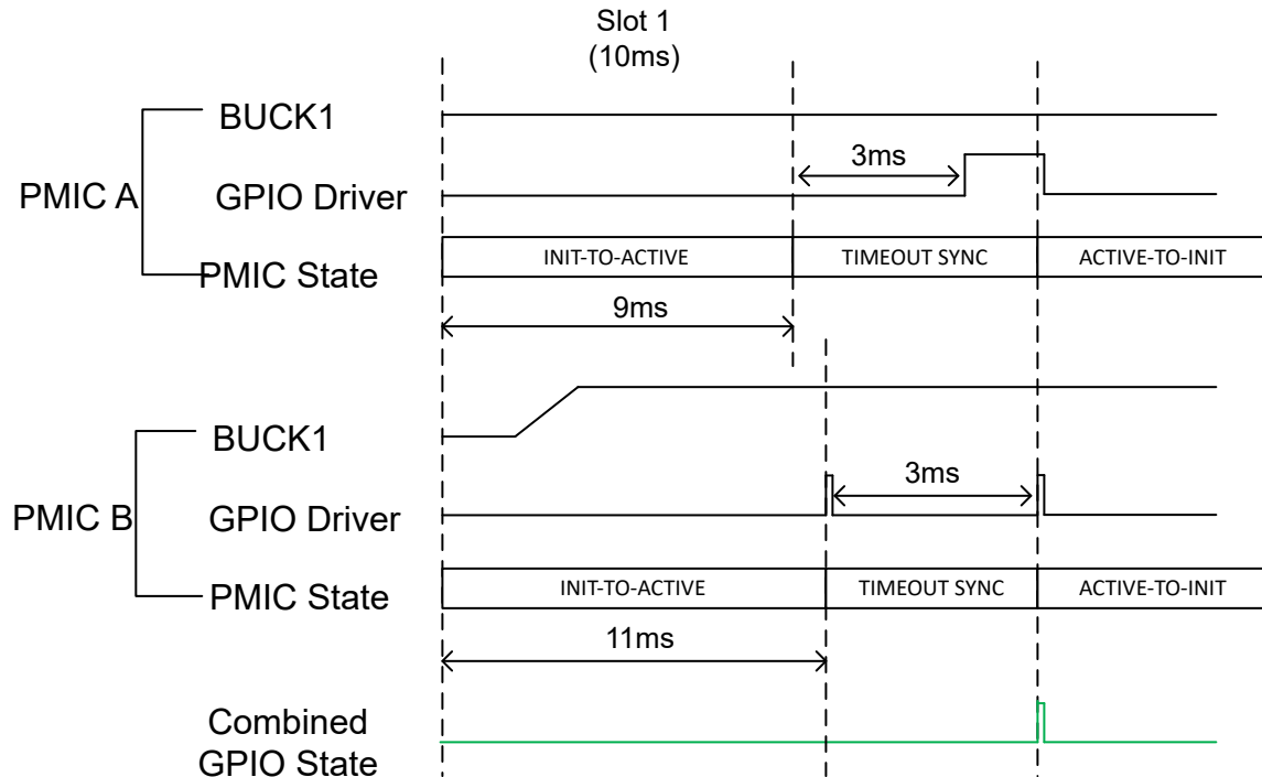
图 7-16. 超时同步
