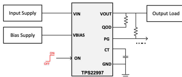
TPS22997 典型应用
