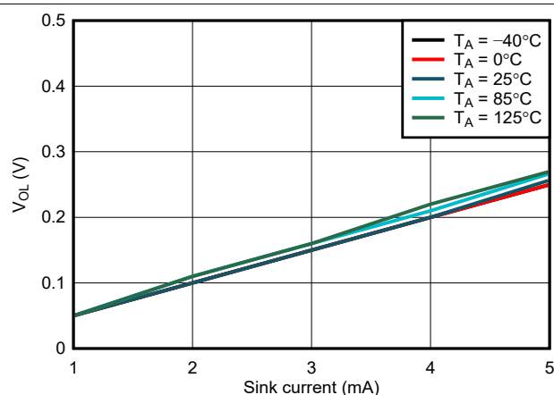
图 7-7. WDO V_{OL} vs I_{sink} , V_{DD} = 3.3\text{ V}
