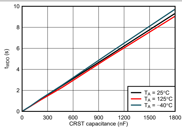
图 7-5. t_{WDO} vs Capacitance
