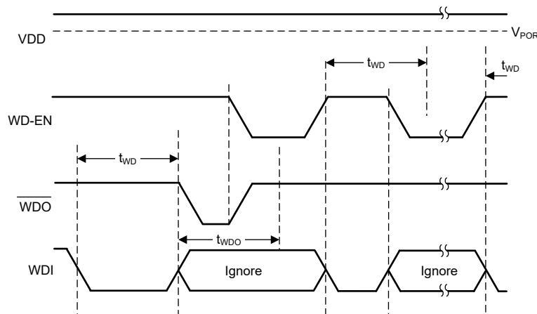
图 8-7. Watchdog Enable: WD-EN Pin Control
