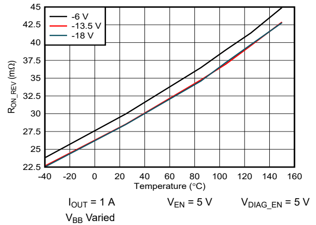
图 6-8. R_{ONREV} vs Temperature
