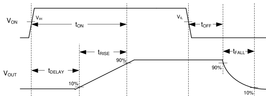
图 7-1. Timing Waveform
