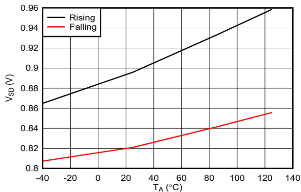
图 6-17. 最低关断电流的 EN/UVLO 引脚阈值与温度间的关系
