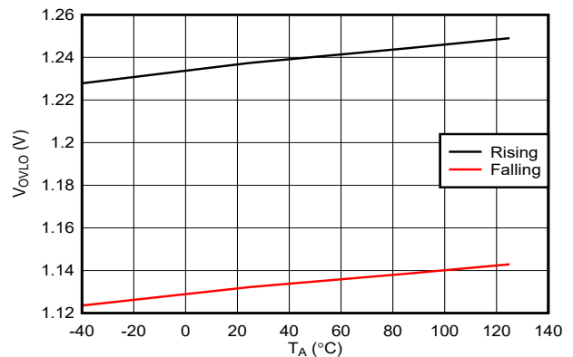
图 6-18. OVLO 引脚阈值与温度间的关系
