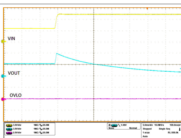
图 8-11. Overvoltage protection
