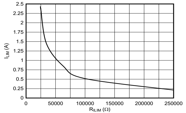
图 6-20. 电流限制阈值与 I_{LIM} 电阻器间的关系
