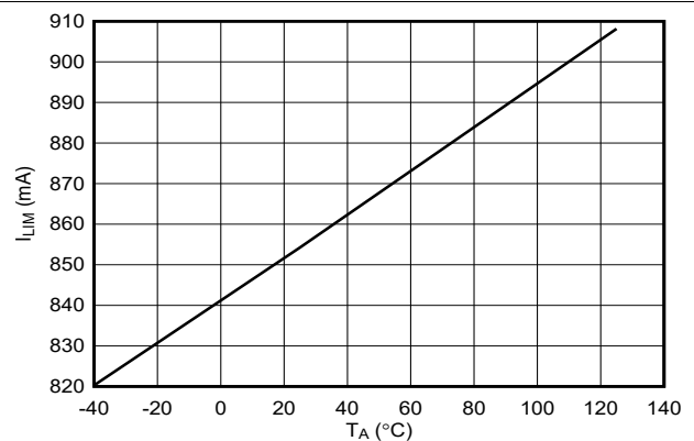
图 6-22. 电流限制阈值与温度间的关系
