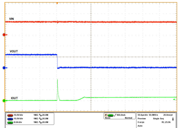
图 6-8. 使用高电流限制设置为大电容器充电 - 断续模式
