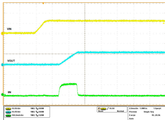
图 6-1. 输入热插拔响应
