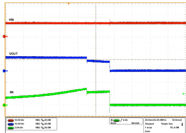
图 6-4. 过压锁定响应 - 可调节阈值
