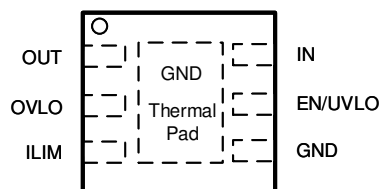
图 5-1. DRV Package, 6-Pin SON (Top View)
