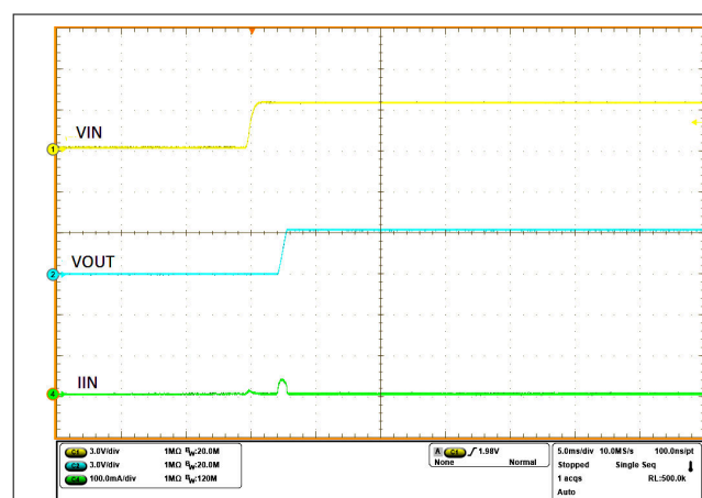
图 8-10. Output Ramp
