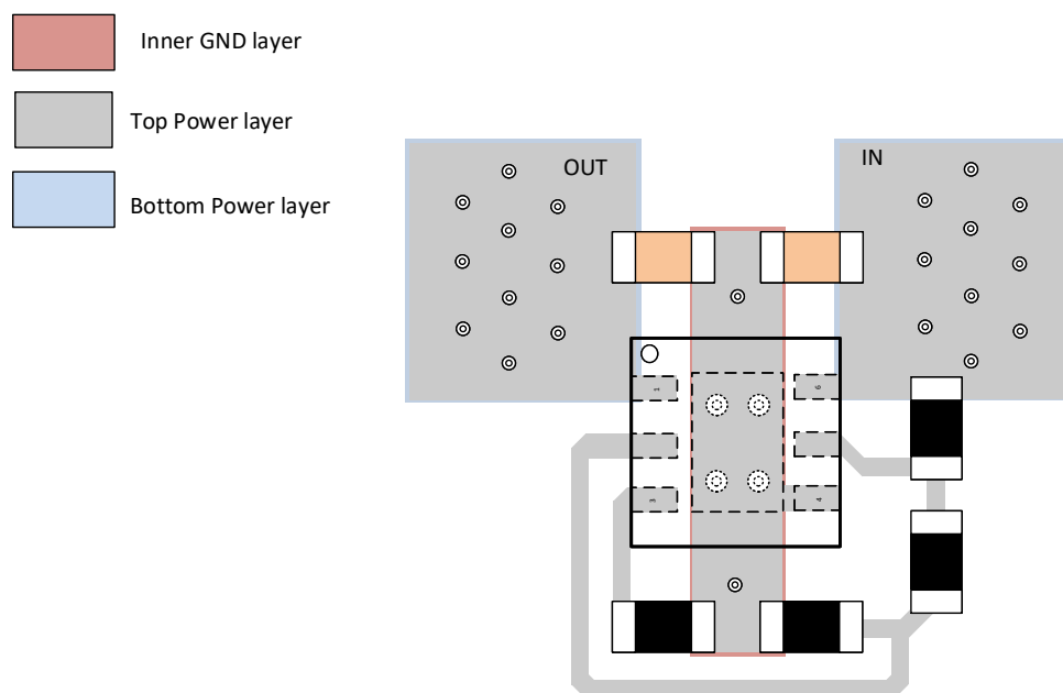
图 8-16. TPS25961 Layout Example
