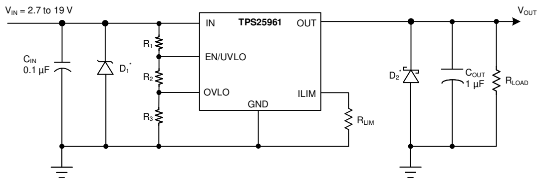
图 8-15. 带有可选保护元件的电路实现
