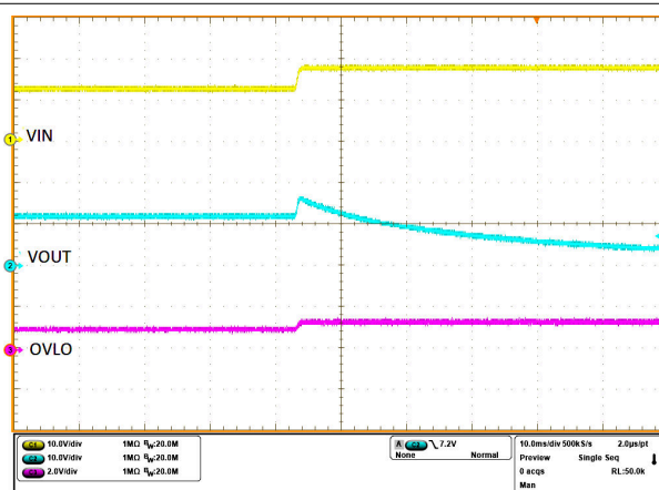
图 8-4. Overvoltage Protection (OVLO)
