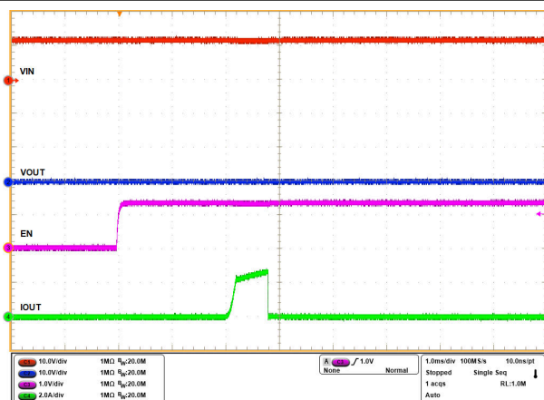
图 6-9. 导通时输出短路
