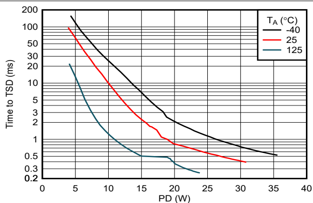
图 6-31. 热关断时间与功率耗散间的关系
