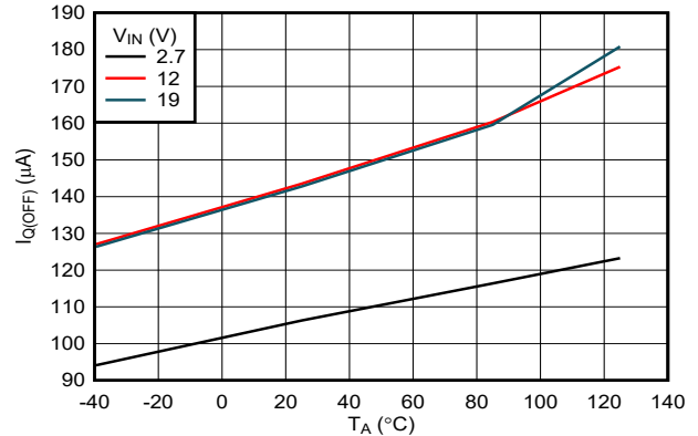
图 6-14. 关断状态电流与温度间的关系
