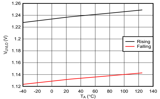
图 6-16. FET 开/关控制的 EN/UVLO 引脚阈值与温度间的关系
