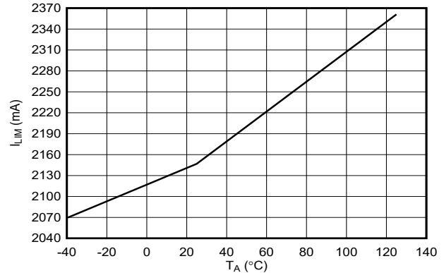
图 6-26. 电流限制阈值与温度间的关系
