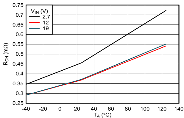
图 6-29. 导通电阻与温度间的关系
