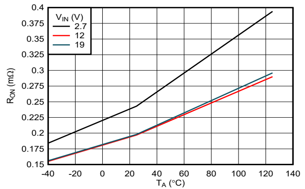
图 6-28. 导通电阻与温度间的关系
