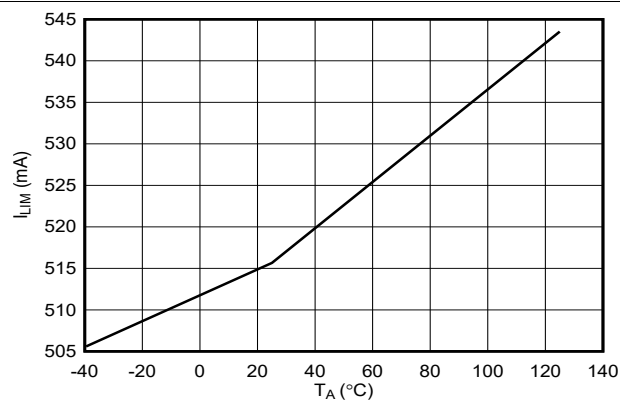
图 6-21. 电流限制阈值与温度间的关系
