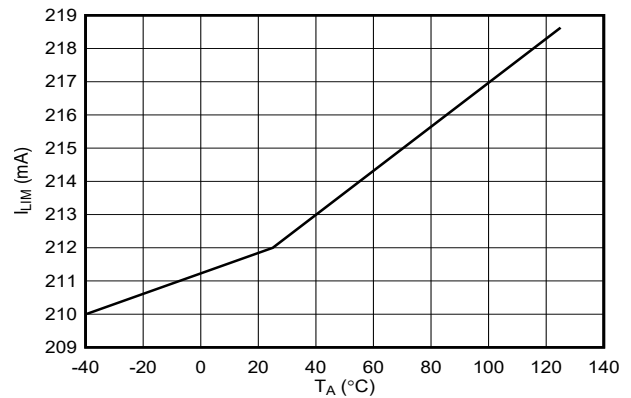
图 6-22. 电流限制阈值与温度间的关系
