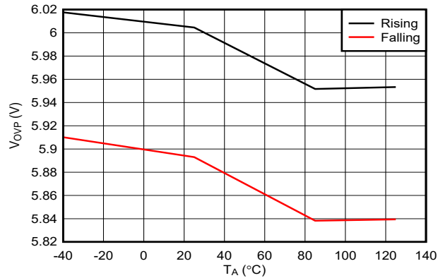
图 6-19. 内部固定过压阈值与温度间的关系
