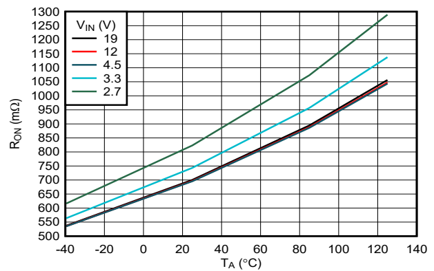
图 6-30. 导通电阻与温度间的关系
