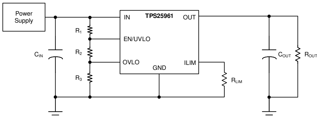
简化原理图
