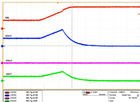
图 6-3. 通过输入电源上电
