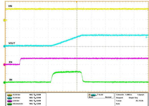
图 6-2. 通过使能引脚上电
