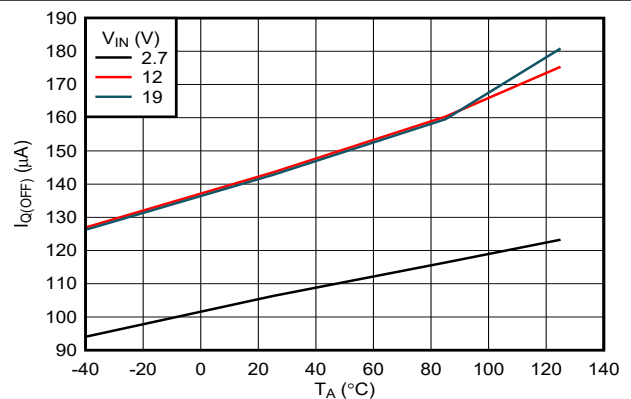
图 6-12. 稳态静态电流与温度间的关系
