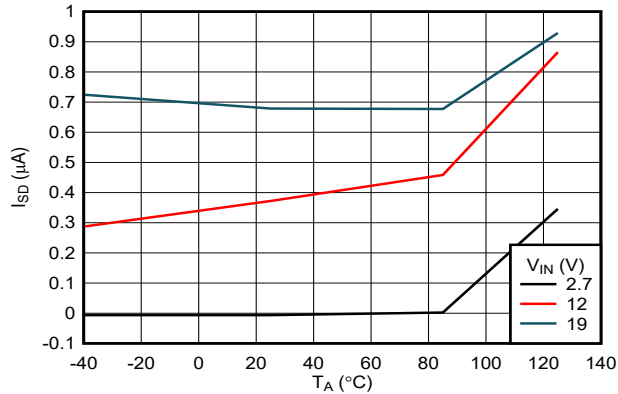
图 6-13. 关断电流与温度间的关系
