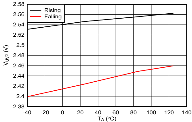
图 6-15. IN 电源欠压阈值与温度间的关系
