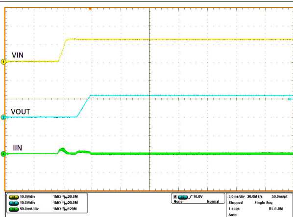
图 8-3. Output Ramp
