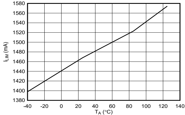
图 6-25. 电流限制阈值与温度间的关系
