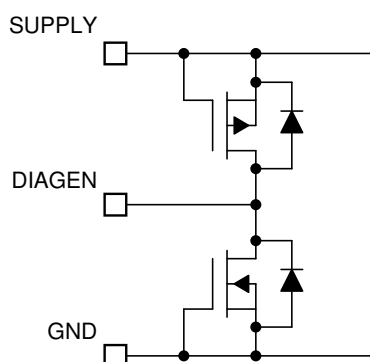
图 6-10. DIAGEN Pin
