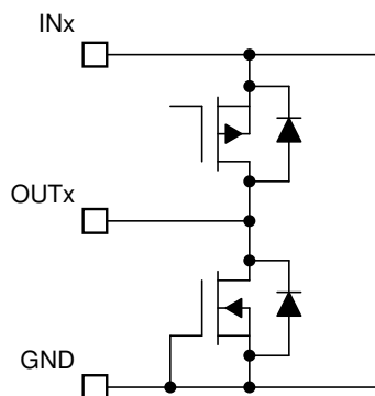
图 6-12. OUTx Pins
