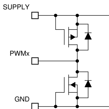
图 6-9. PWMx Pins
