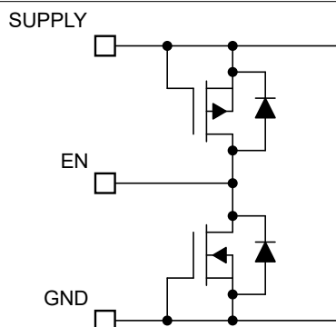
图 6-8. EN Pin
