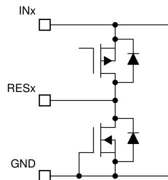
图 6-13. RESx Pins
