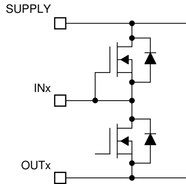
图 6-14. INx Pins
