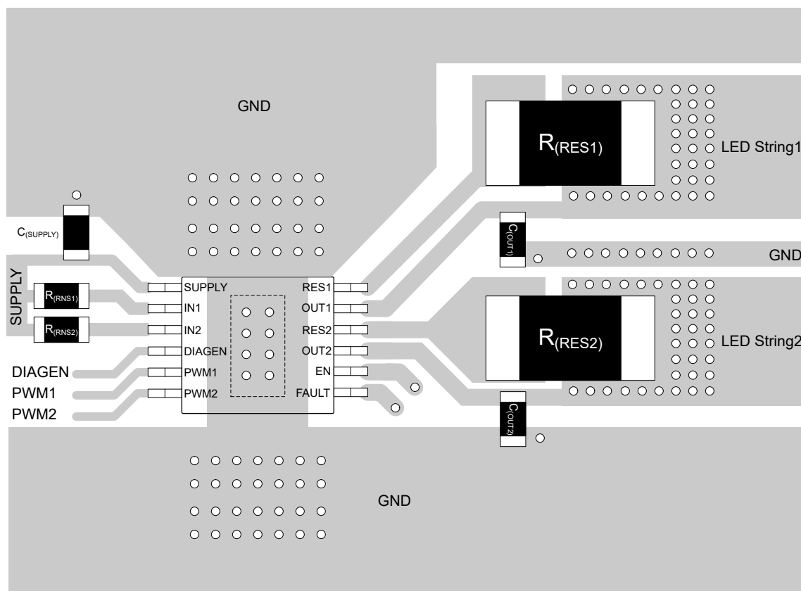
图 7-7. TPS92622-Q1 Example Layout Diagram
