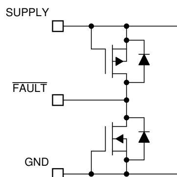
图 6-11. FAULT Pin
