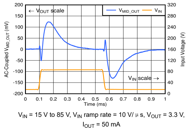
图 6-16. Line Transient
