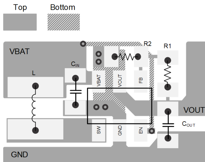
图 8-13. PCB Layout
