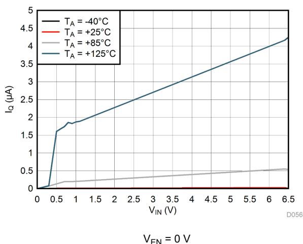
图 6-16. LP5912-3.3 I_{Q(SD)} vs V_{IN}
