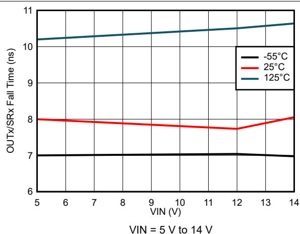
图 7-60. Output Fall Time Variation
