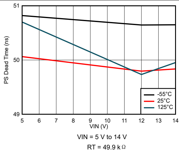
图 7-44. PS Dead Time Variation
