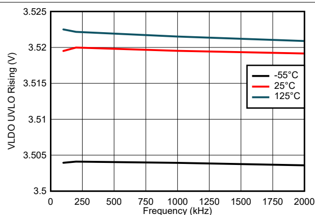
图 7-5. VLDO UVLO Rising Variation
