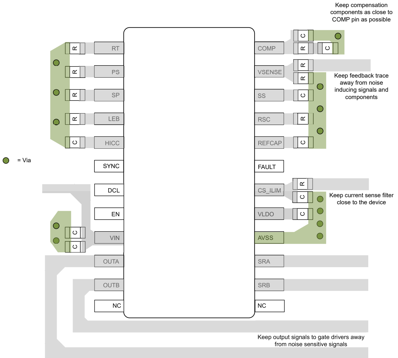
图 11-1. PCB Layout Example
