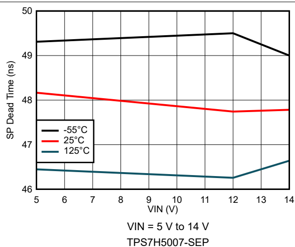
图 7-56. SP Dead Time Variation
