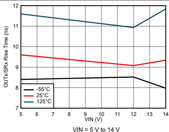
图 7-58. Output Rise Time Variation
