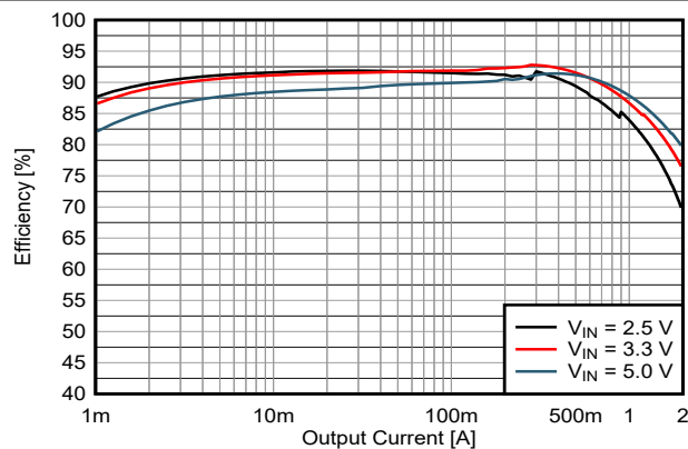
图 8-17. 1.2V Output Efficiency
