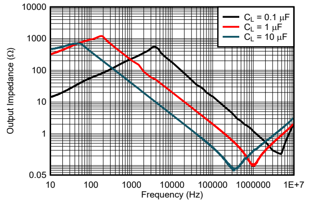
图 6-32. Output Impedance
