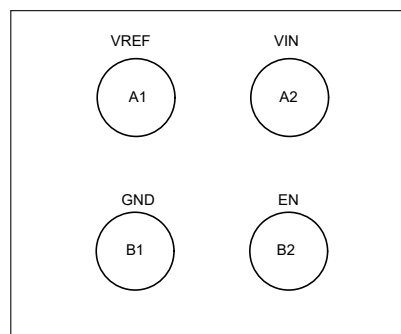
图 5-2. YBH Package 4-Pin WCSP Top View
