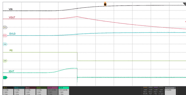
图 8-9. Overvoltage Response
