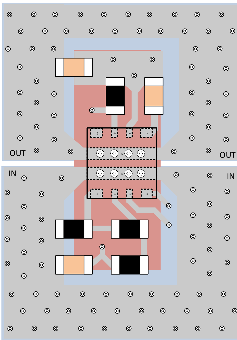
图 10-1. Layout Example
