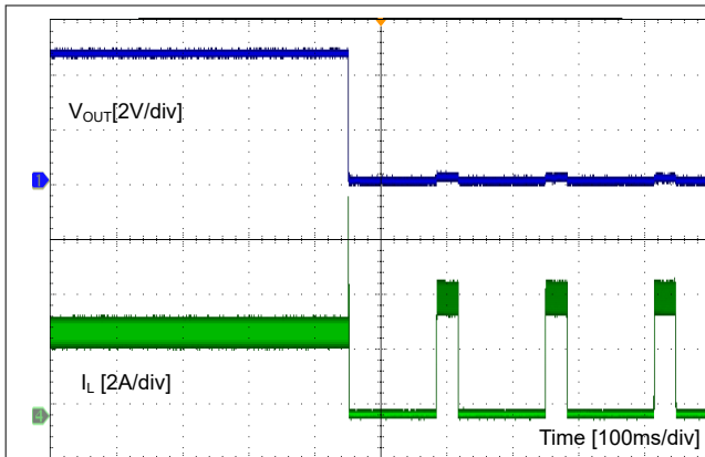
图 9-8. Short Protection
