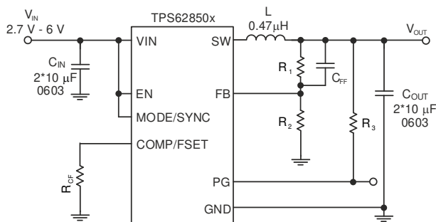
简化原理图
