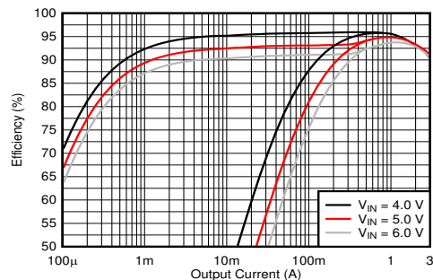
效率与 I_{OUT} 间的关系， V_{OUT} = 3.3V
