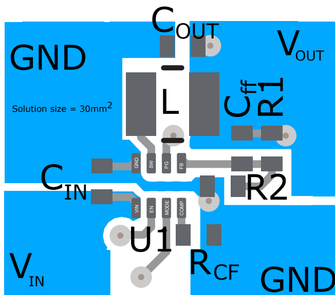
图 9-60. Example Layout
