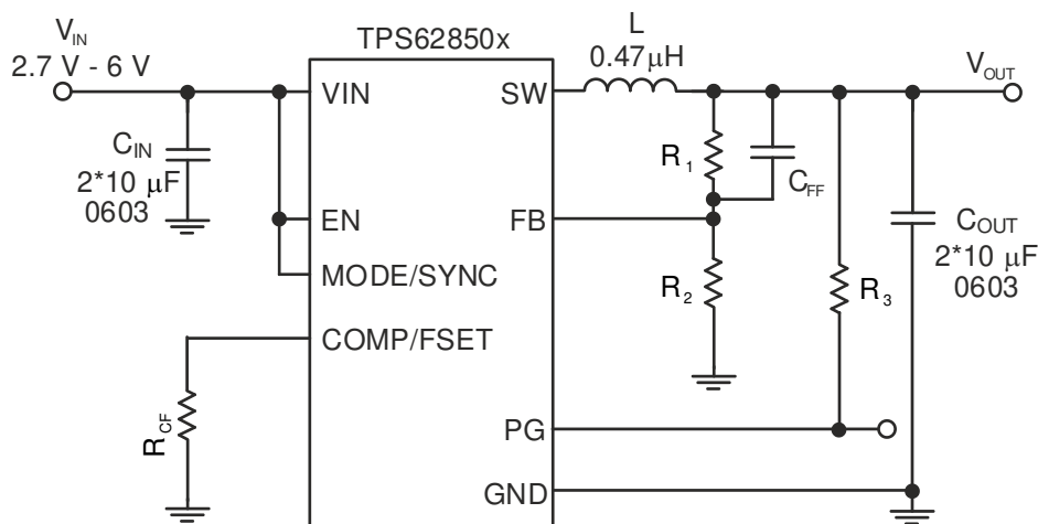
图 7-1. Measurement Setup
