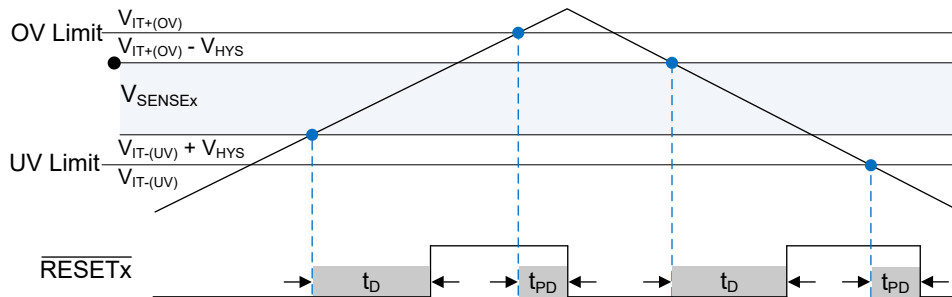
图 7-6. RESETx Output
