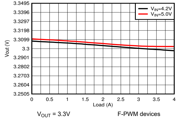
图 8-22. Load Regulation
