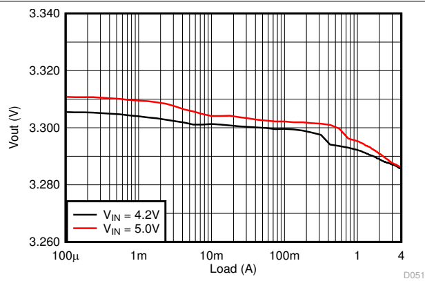
图 8-20. Load Regulation
