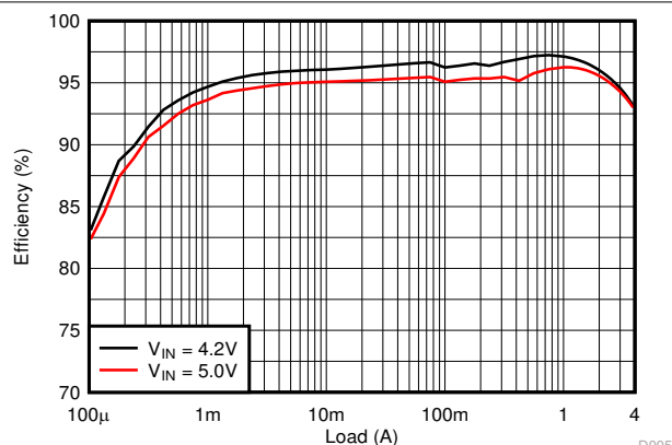
图 8-17. PWM Efficiency
